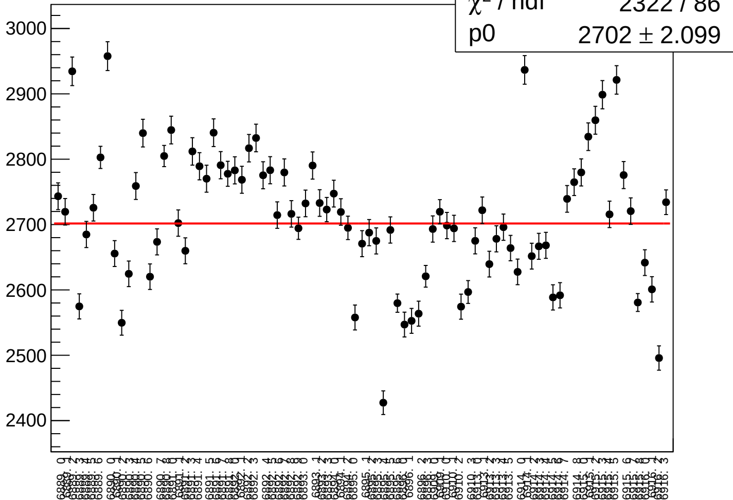
\chi^2 / \text{ndf}
