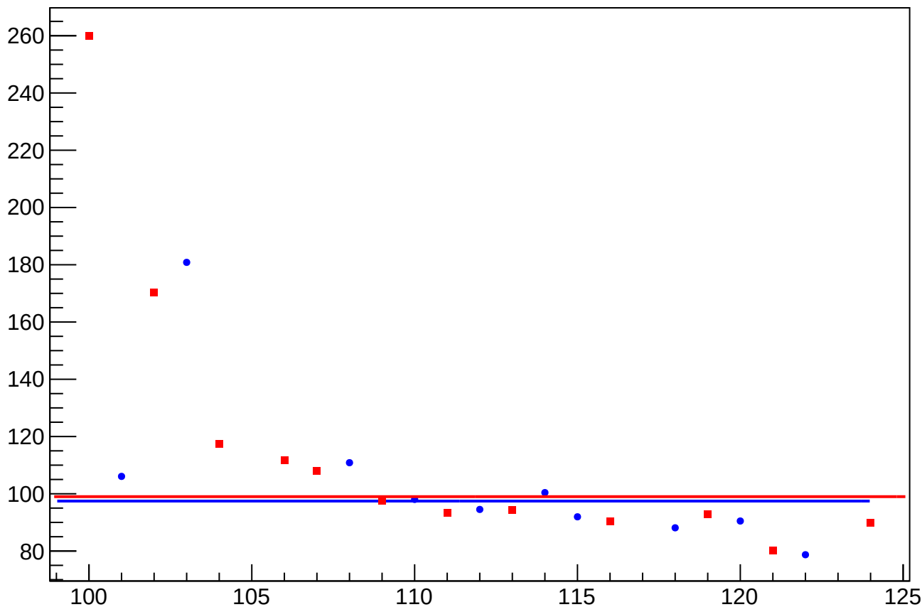
cor_asym_sam_2468_avg_rms vs Slug
