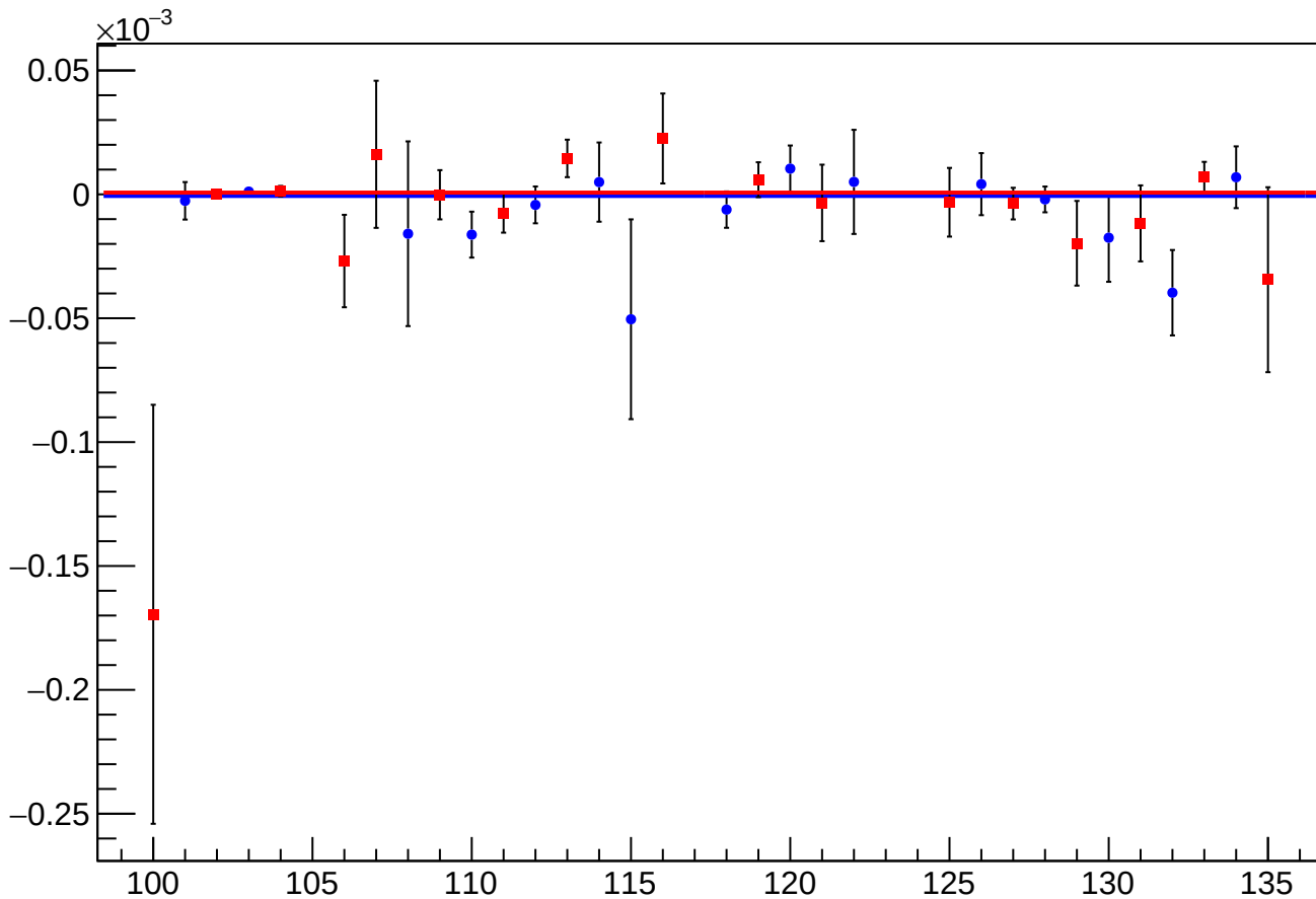
asym us dd at2lr dd dd eigen dit vs dit diff mean vs Slug
