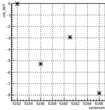
usl_4aY:cyclenum
