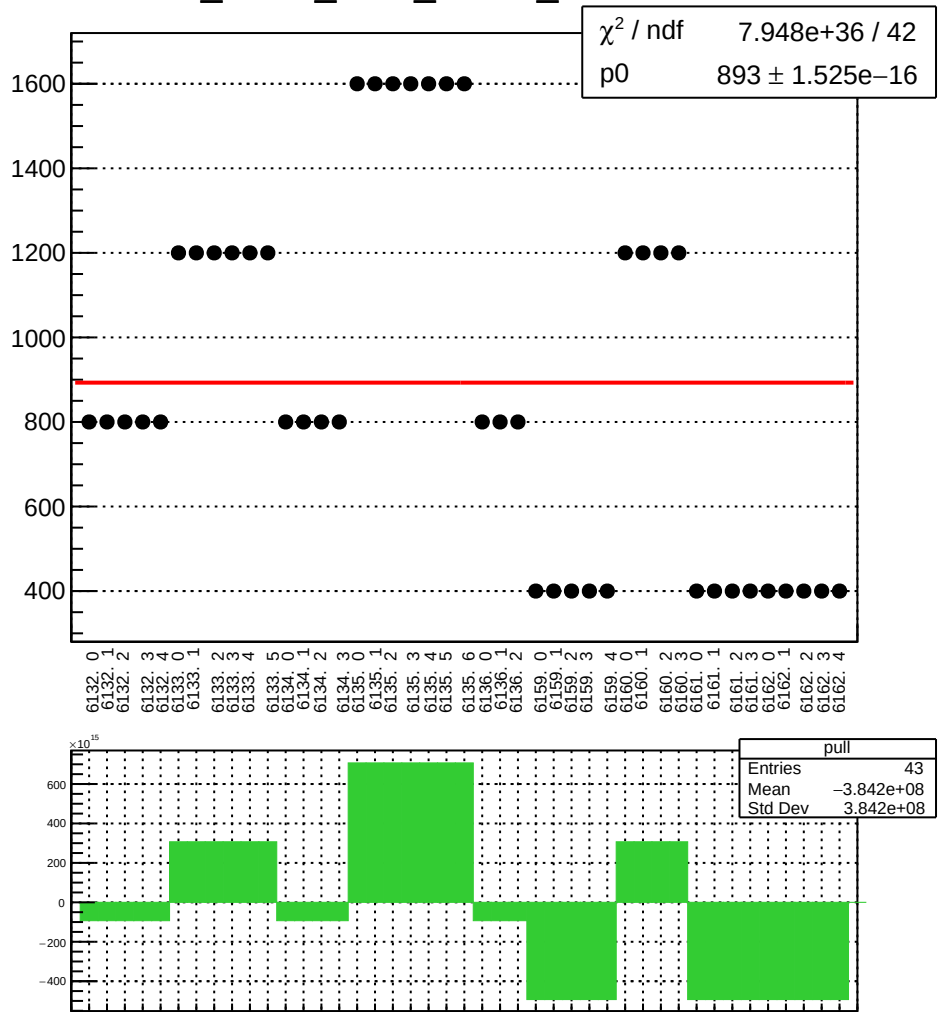
dit_sam3_coil3_Ndata_mean vs run
