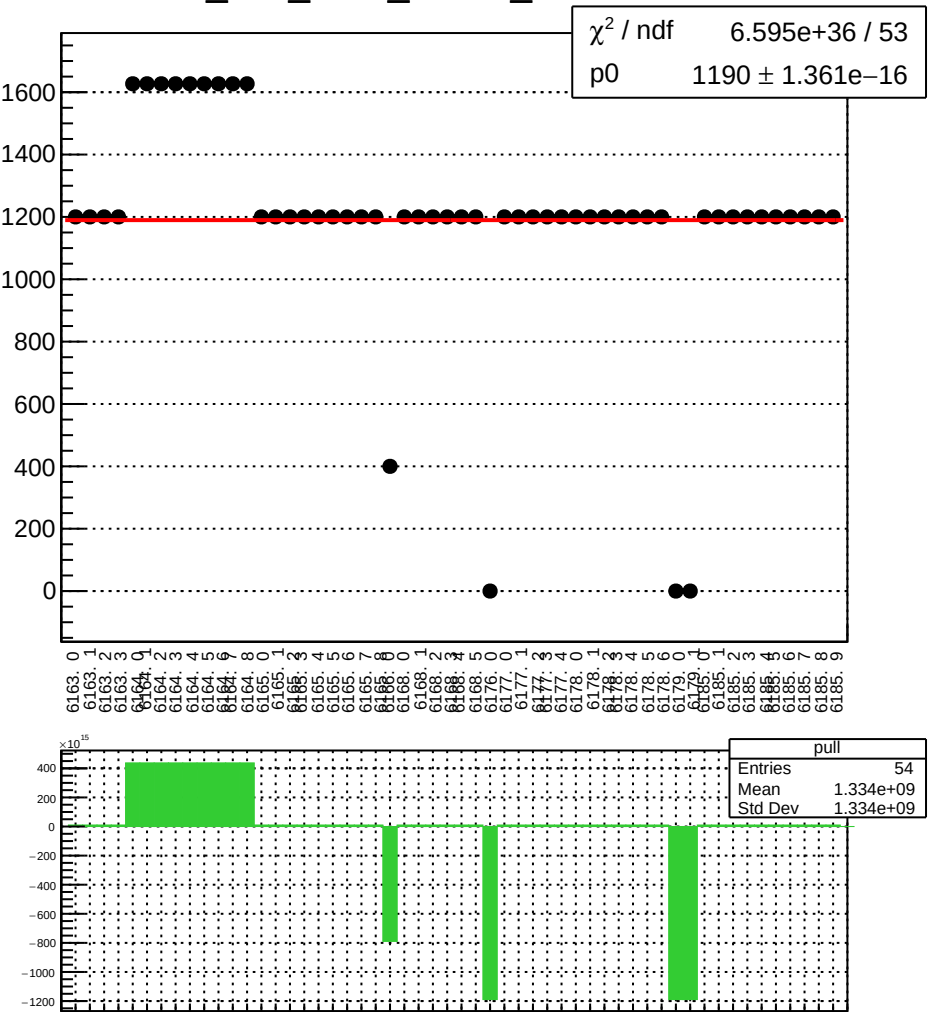
dit_atl1_coil3_Ndata_mean vs run
