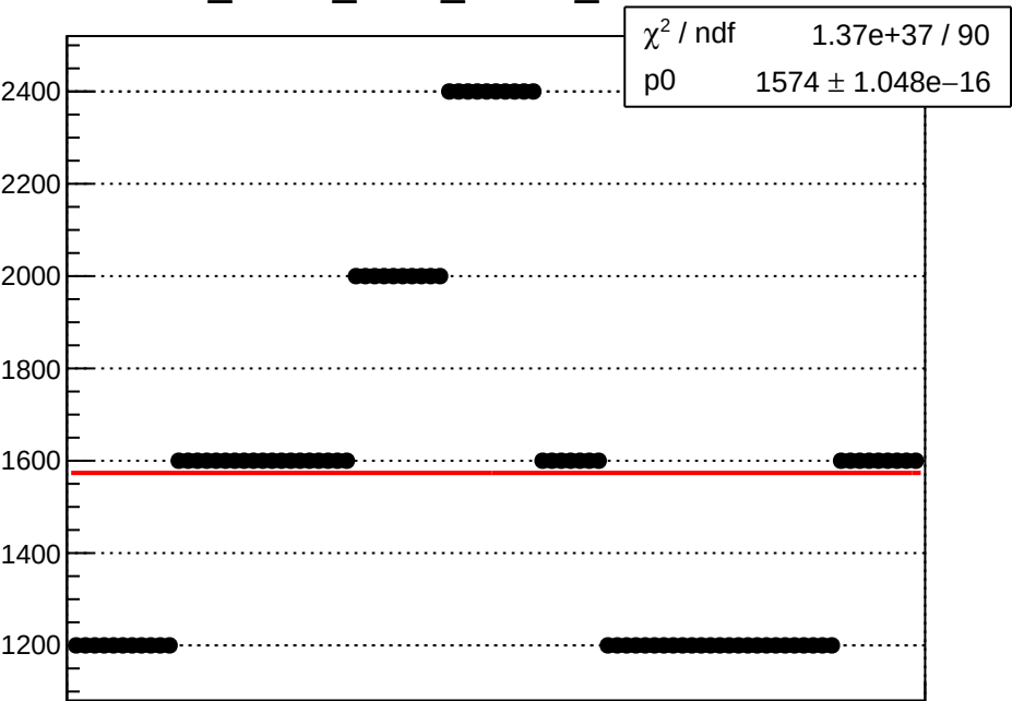
dit_sam1_coil4_Ndata_mean vs run
