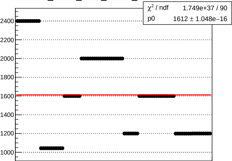
dit_sam2_coil6_Ndata_mean vs run
