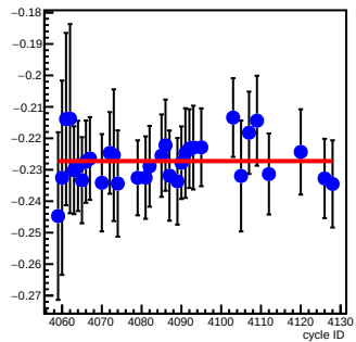
bpm4aX_coil7(um/count)
