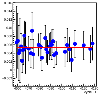
bpm4eY_coil7(um/count)
