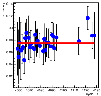
bpm4aX_coil7(um/count)
