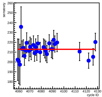
atr2_coil7(ppm/count)
