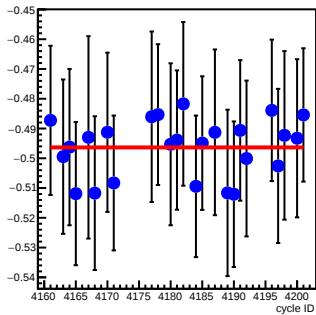
bpm12X_coil7(um/count)
