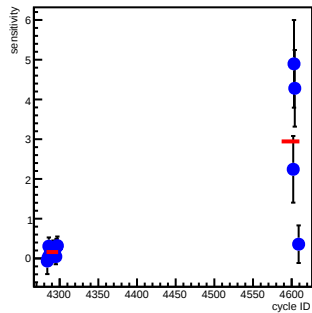
sam5_coil7(ppm/count)
