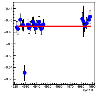
bpm12X_coil7(um/count)
