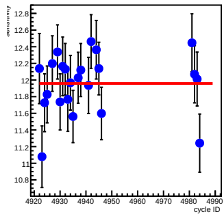
usl_coil7(ppm/count)
