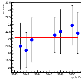
at12_coil7(ppm/count)
