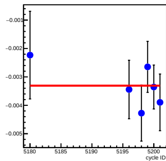
bpm4eY_coil5(um/count)
