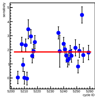
usl_coil7(ppm/count)
