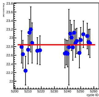
usl_coil7(ppm/count)
