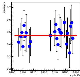
sam7_coil6(ppm/count)
