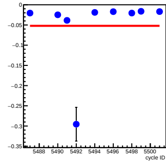
bpm4aY_coil7(um/count)
