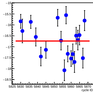
sam6_coil7(ppm/count)
