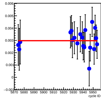
bpm4eY_coil7(um/count)
