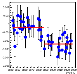
bpm4eY_coil5(um/count)
