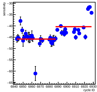
sam6_coil7(ppm/count)
