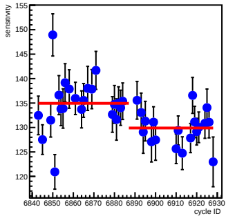
at12_coil7(ppm/count)
