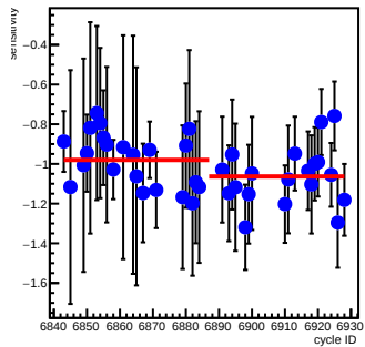
sam8_coil7(ppm/count)
