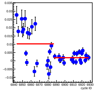
bpm4eX_coil6(um/count)
