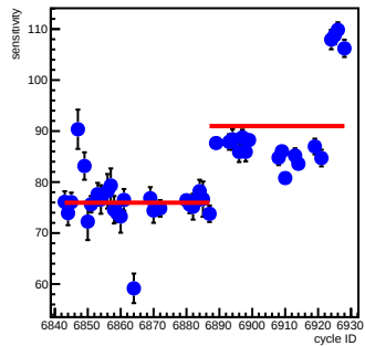
sam2_coil7(ppm/count)
