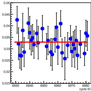
bpm4eX_coil7(um/count)
