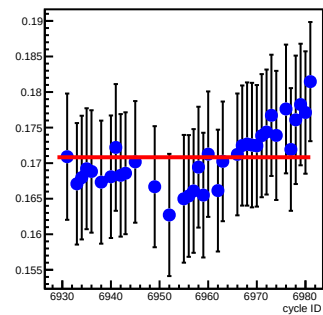
bpm4eX_coil5(um/count)
