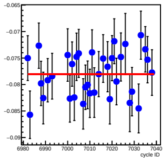
bpm12X_coil2(um/count)
