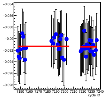
bpm4eX_coil2(um/count)
