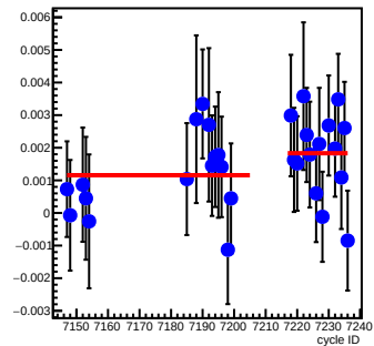
bpm4eX_coil6(um/count)
