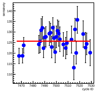
atr2_coil7(ppm/count)
