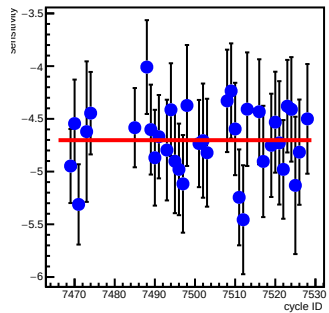
sam5_coil7(ppm/count)
