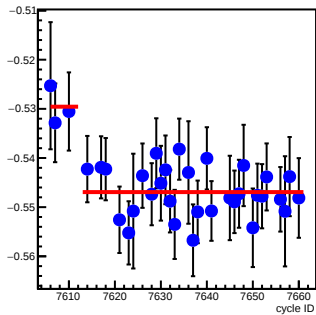
bpm4aX_coil7(um/count)
