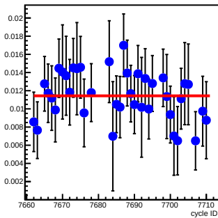
bpm4eX_coil2(um/count)
