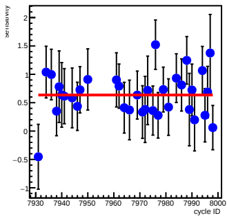
sam6_coil7(ppm/count)
