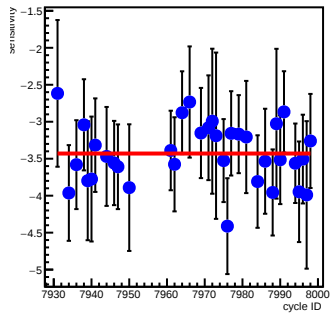
sam3_coil7(ppm/count)
