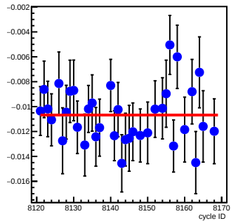
bpm4eY_coil7(um/count)
