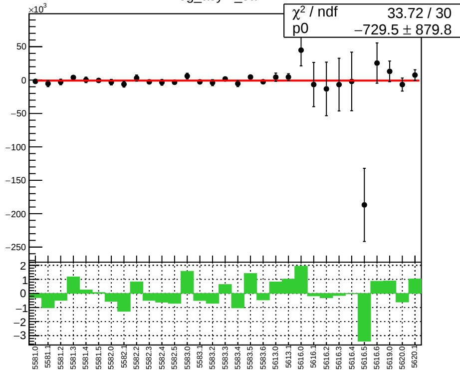
reg_asym_sam2
