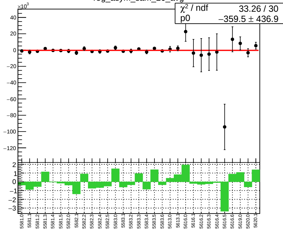
reg_asym_sam_26_avg
