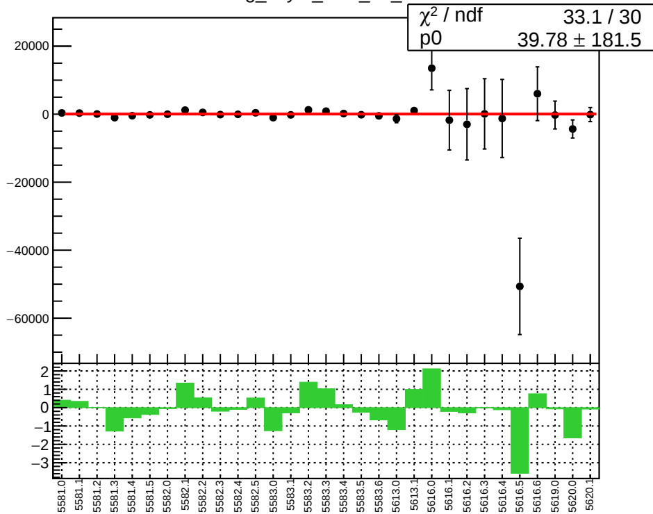
reg_asym_sam_48_dd
