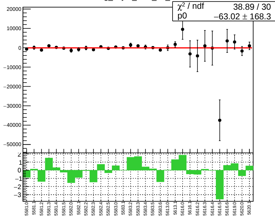
reg_asym_sam_37_dd
