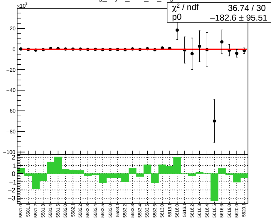
reg_asym_sam_15_avg
