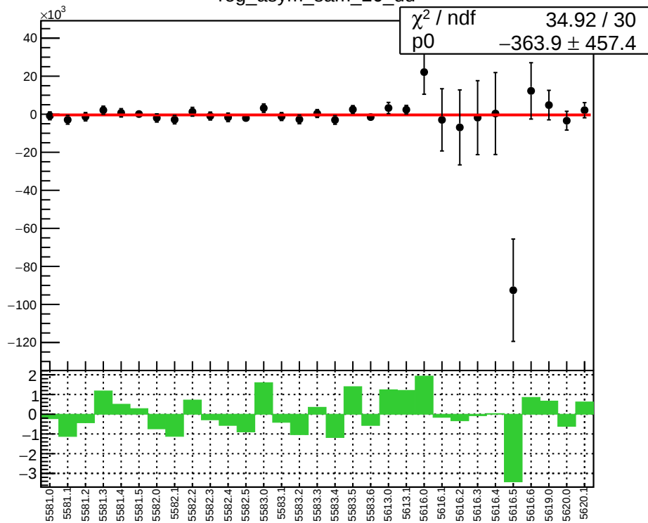
reg_asym_sam_26_dd
