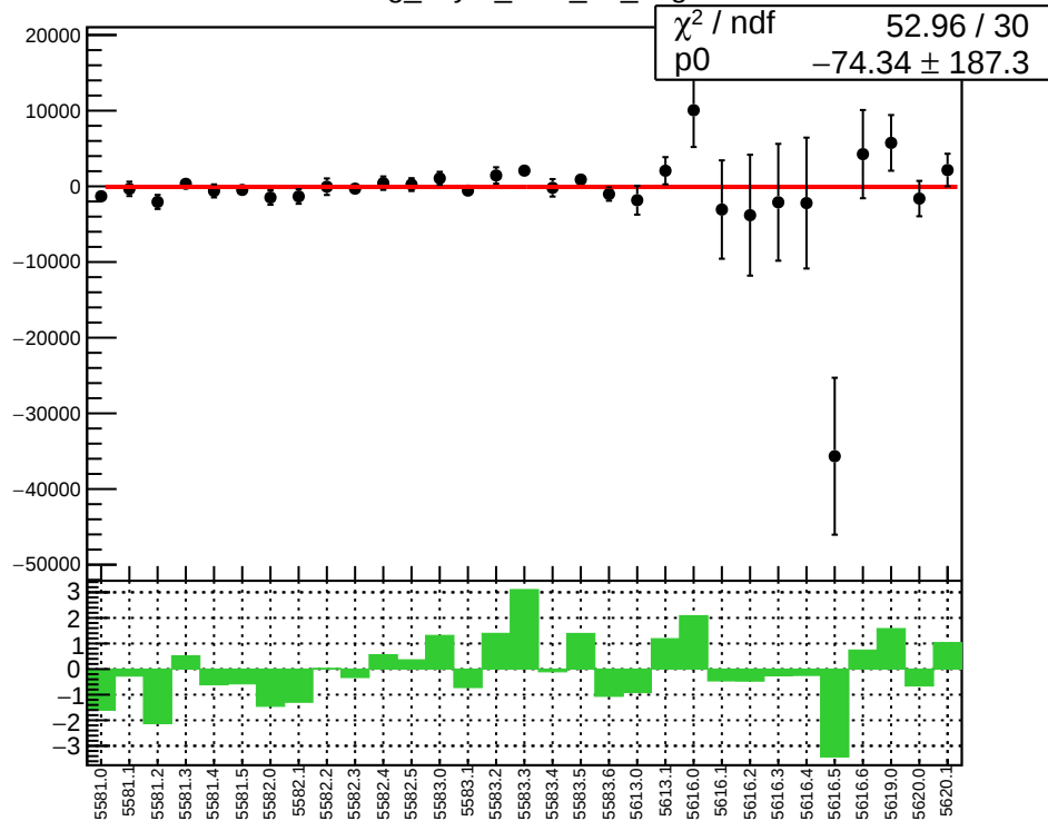
reg_asym_sam_37_avg
