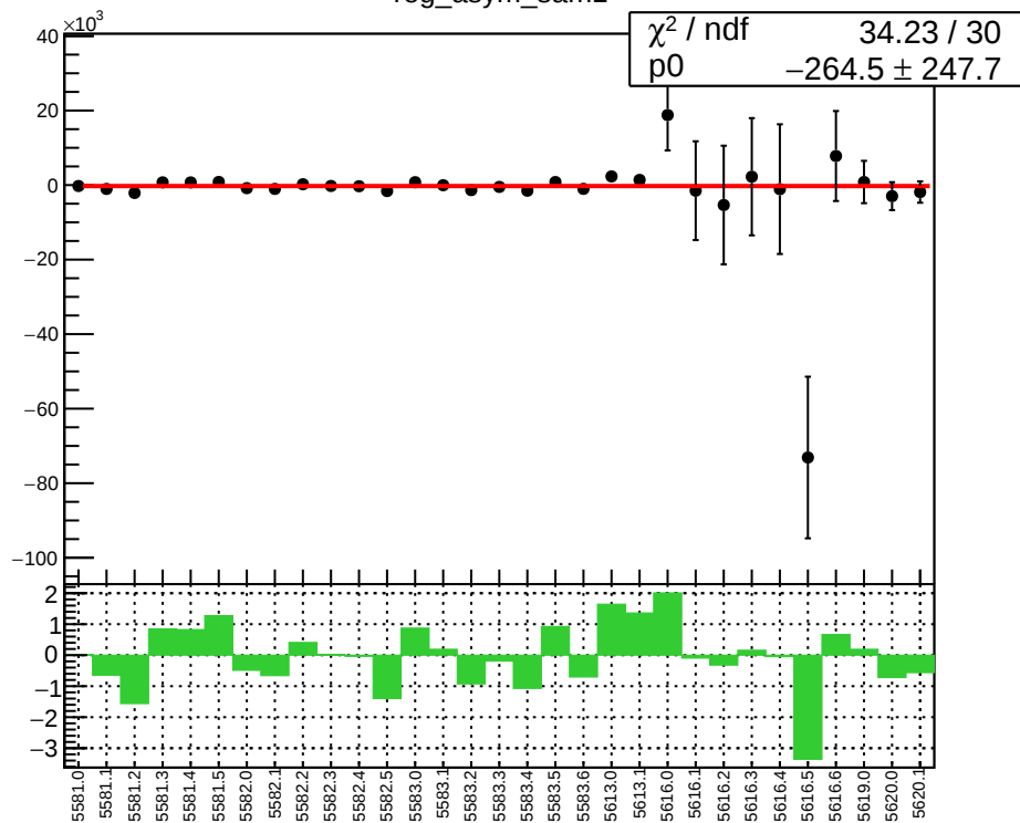
reg_asym_sam1
