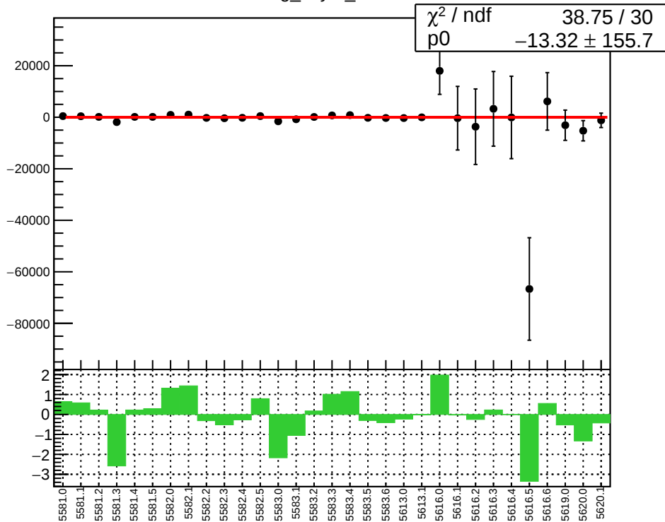
reg_asym_sam5
