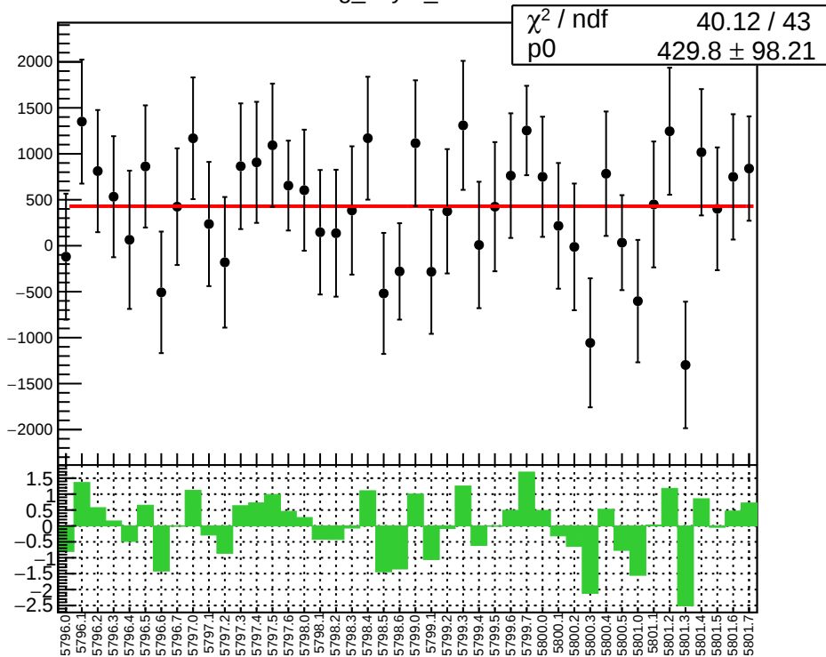
reg_asym_sam8
