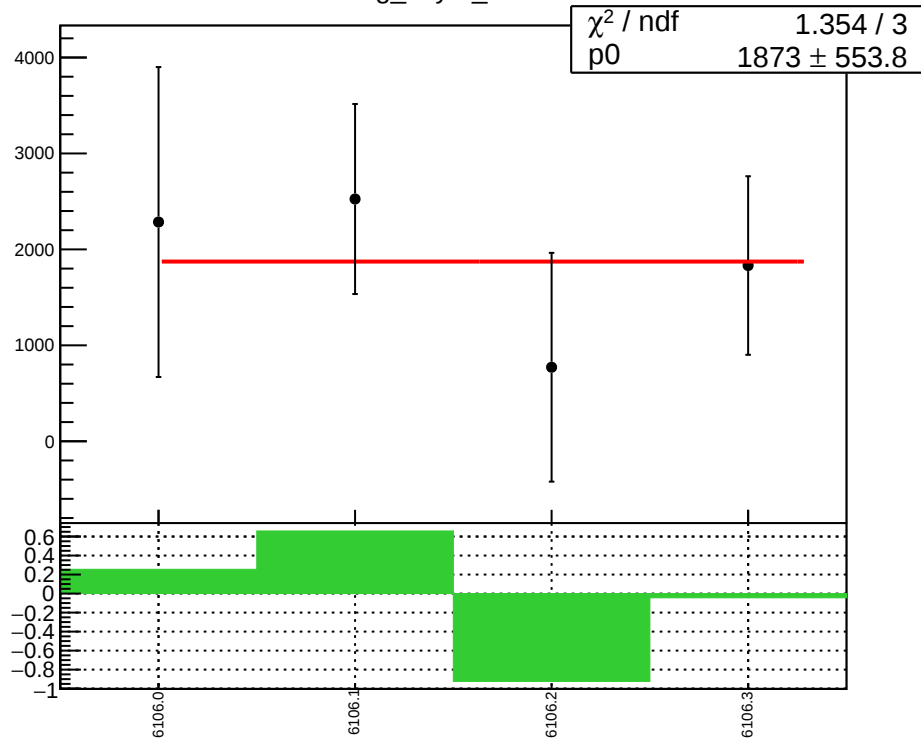
reg_asym_sam3
