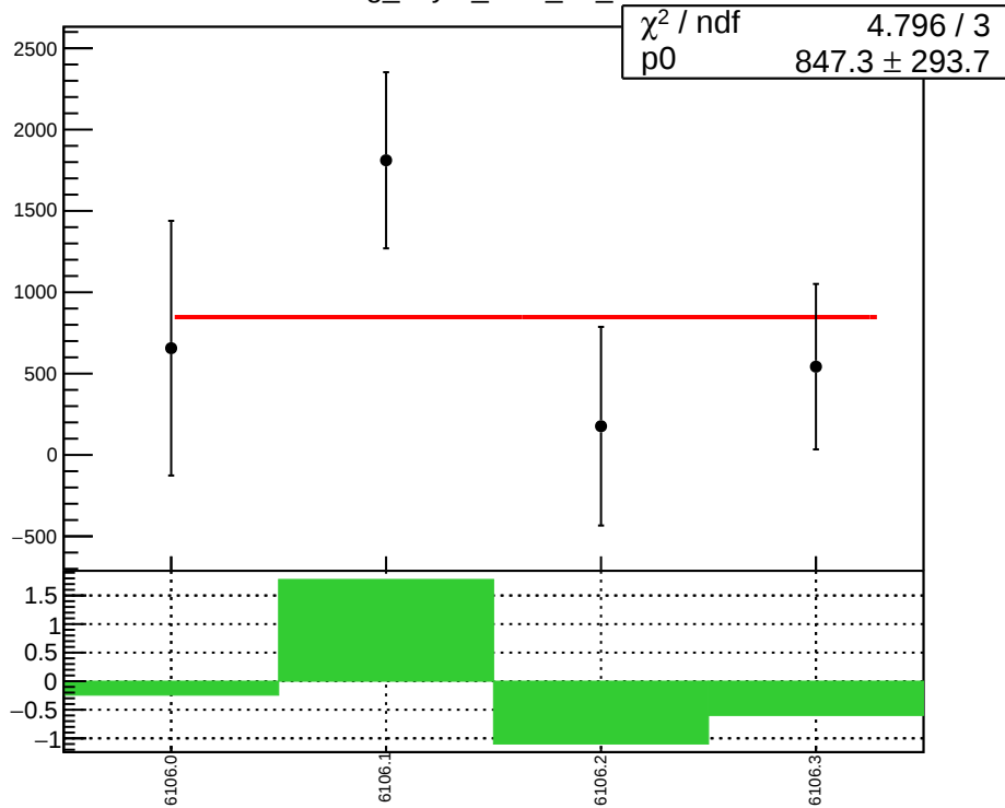
reg_asym_sam_37_dd
