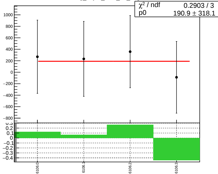
reg_asym_sam_15_avg
