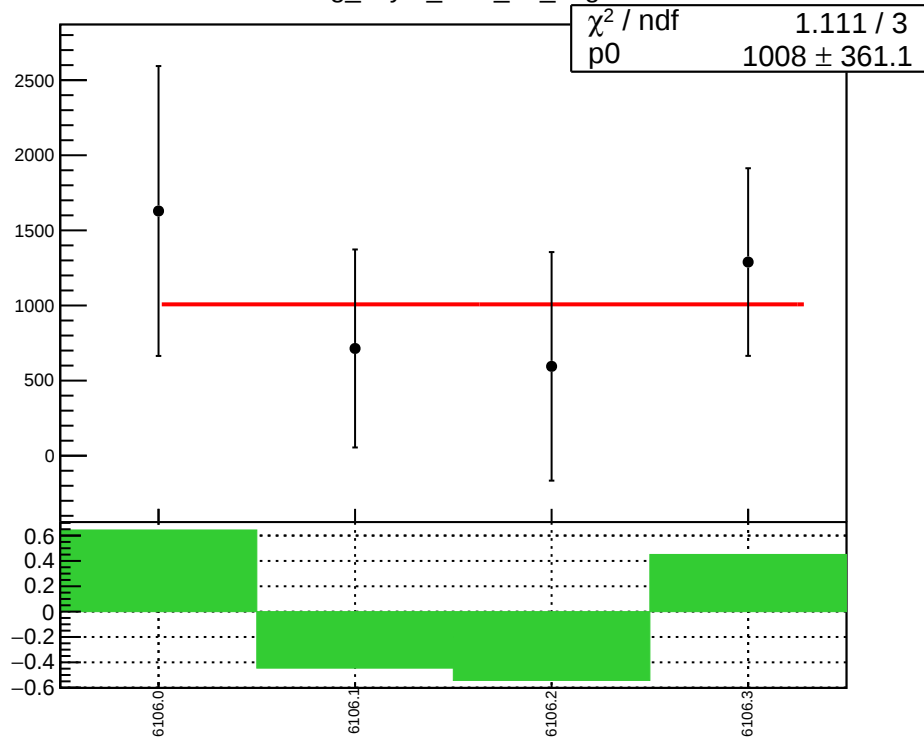
reg_asym_sam_37_avg
