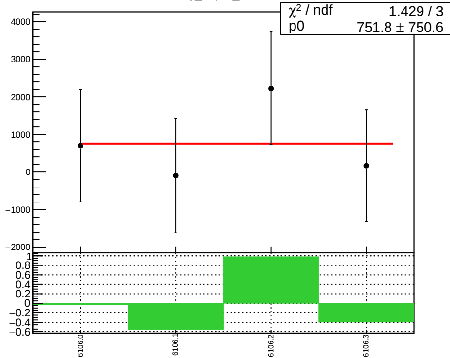
reg_asym_sam5
