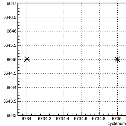
run:cyclenum {run == 6645}
