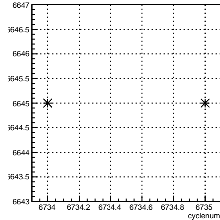
run:cyclenum {run == 6645}
