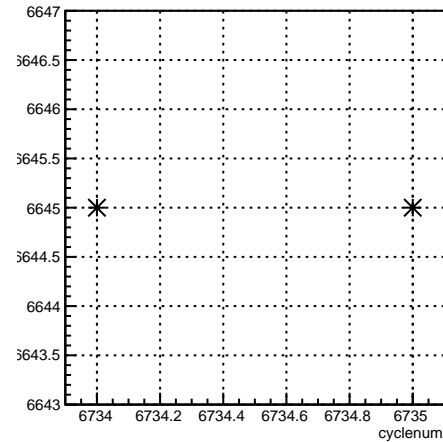
run:cyclenum {run == 6645}
