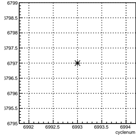
run:cyclenum {run == 6797}
