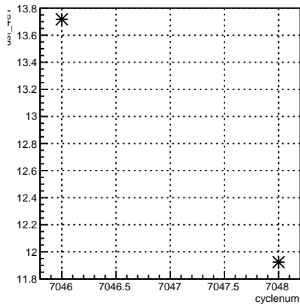
usr_4eY:cyclenum {run == 6808}
