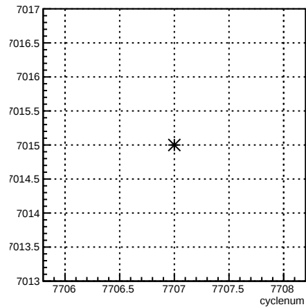
run:cyclenum {run == 7015}
