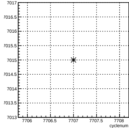
run:cyclenum {run == 7015}
