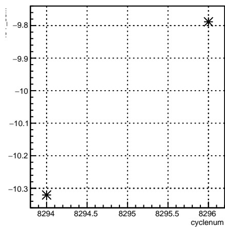
4eY_coil7:cyclenum {run == 7185}
