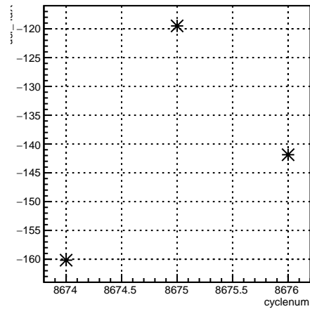
usr_4eY:cyclenum {run == 7315}
