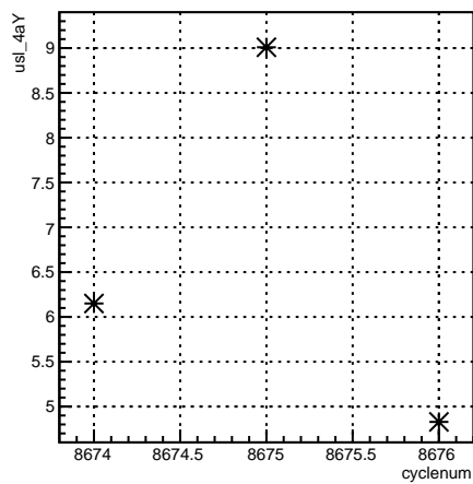
usl_4aY:cyclenum {run == 7315}
