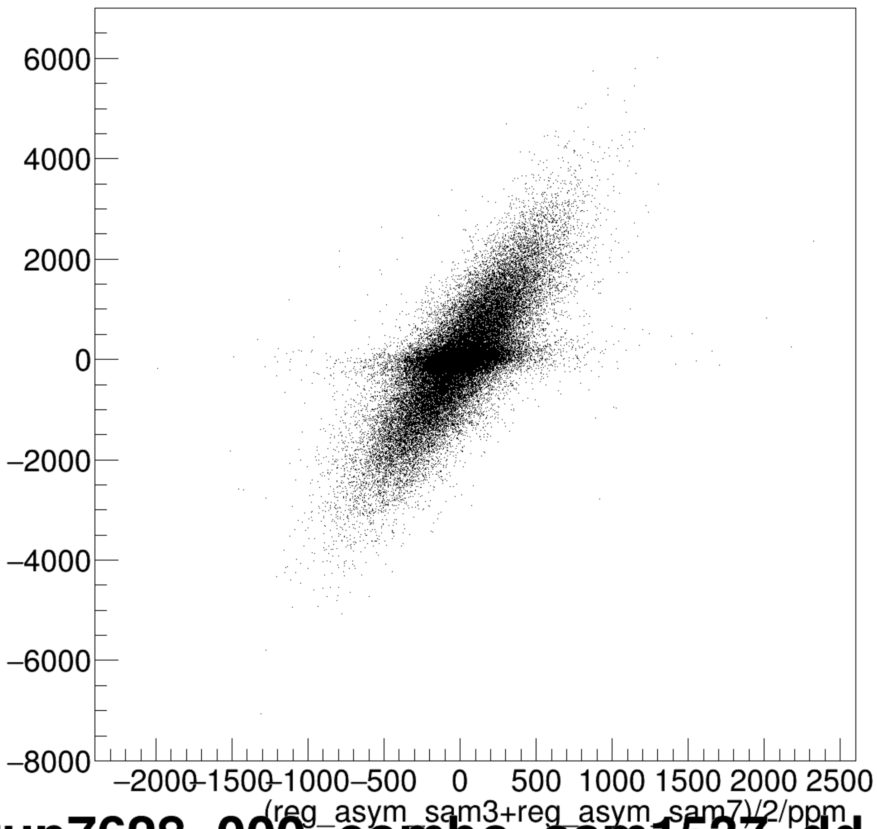
(reg_asym_sam1+reg_asym_sam5)/2/ppm:(reg_asym_sam3+reg_asym_sam7)/2/ppm {ok_cut}
