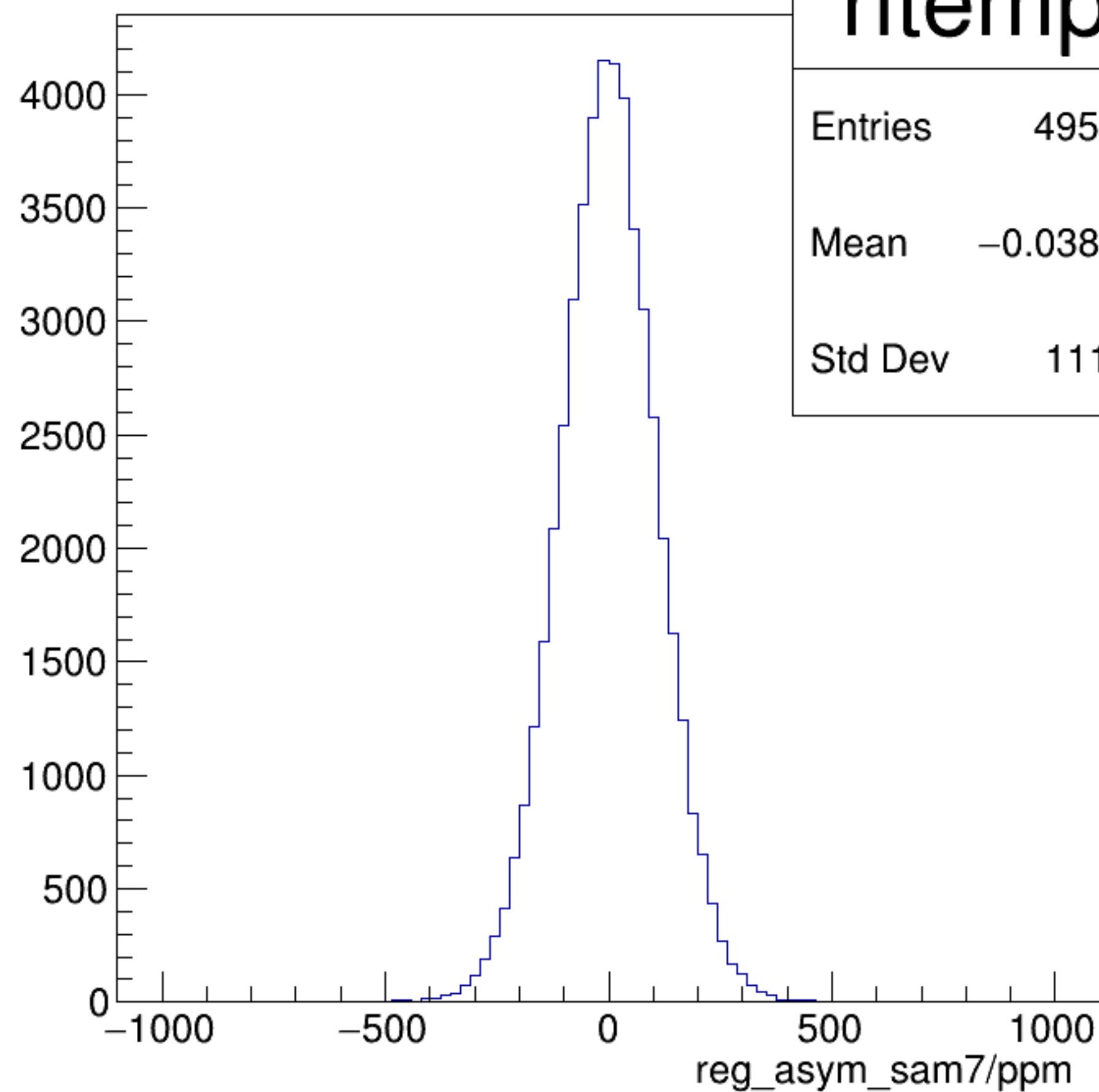
reg_asym_sam7/ppm {ok_cut}
