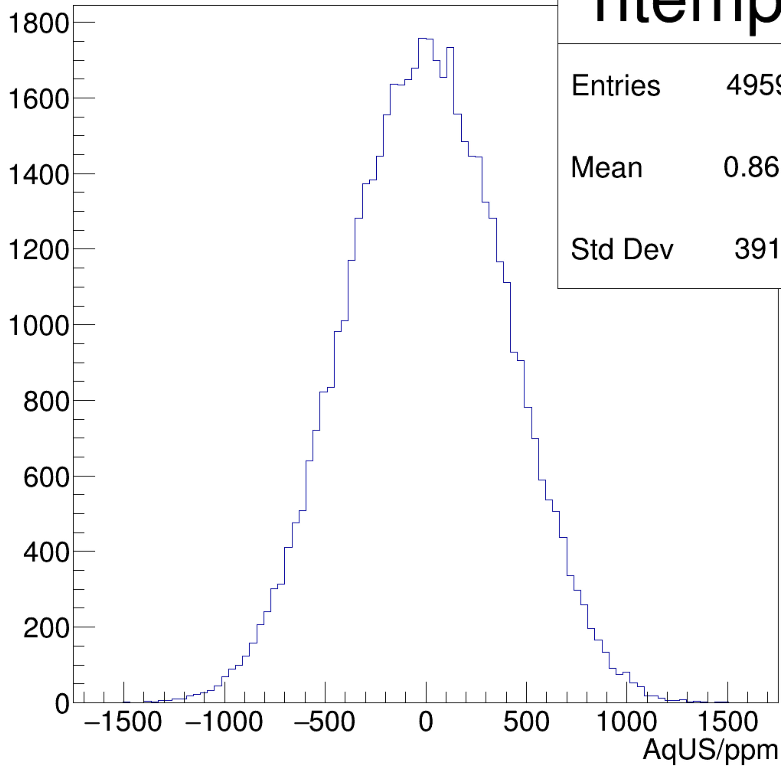
AqUS/ppm {ok_cut}
