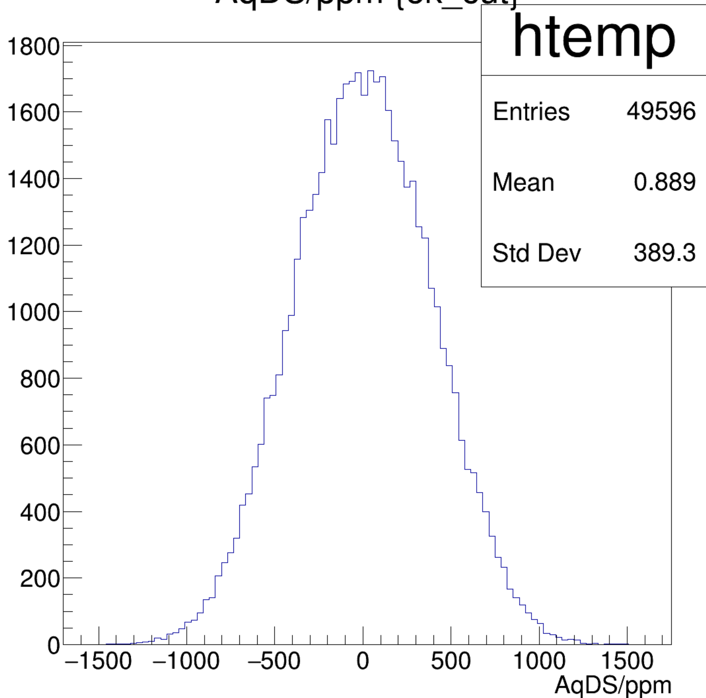
AqDS/ppm {ok_cut}
