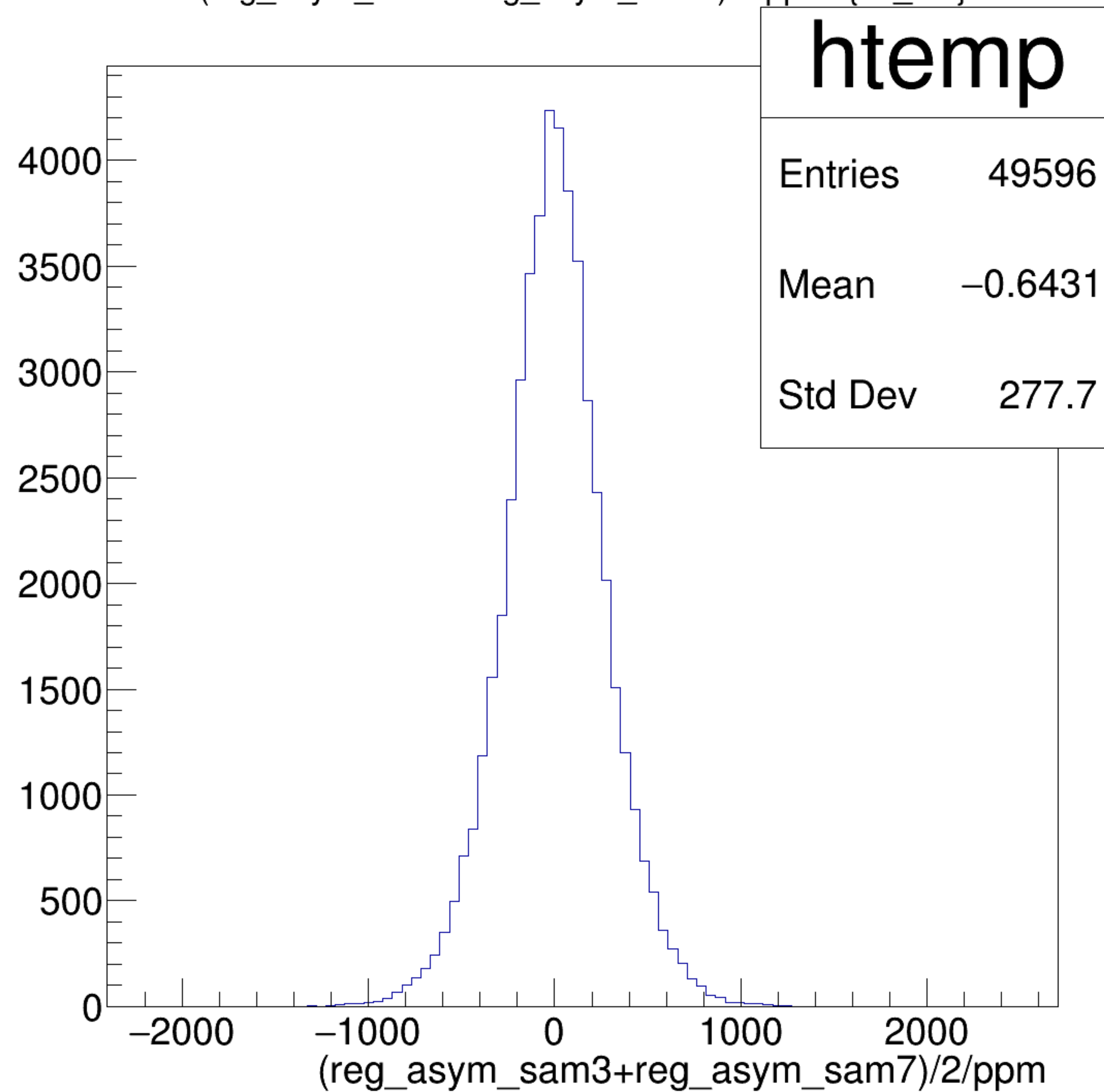
(reg_asym_sam3+reg_asym_sam7)/2/ppm {ok_cut}
