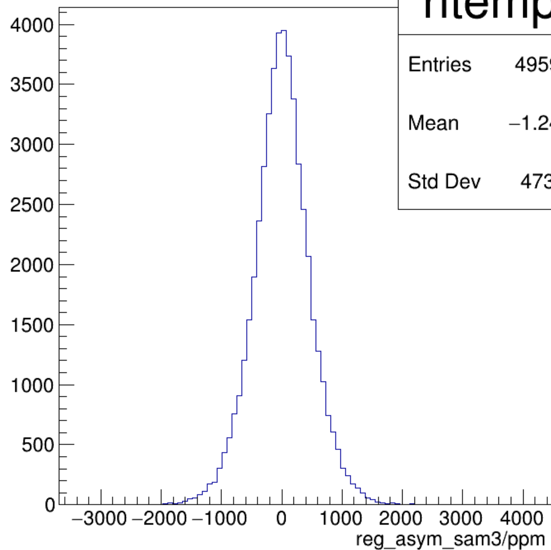
reg_asym_sam3/ppm {ok_cut}
