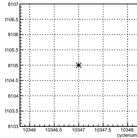
run:cyclenum {run == 8105}
