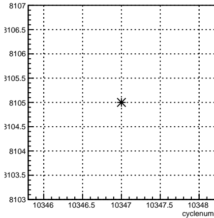
run:cyclenum {run == 8105}
