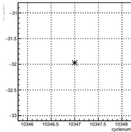
4eY_coil7:cyclenum {run == 8105}
