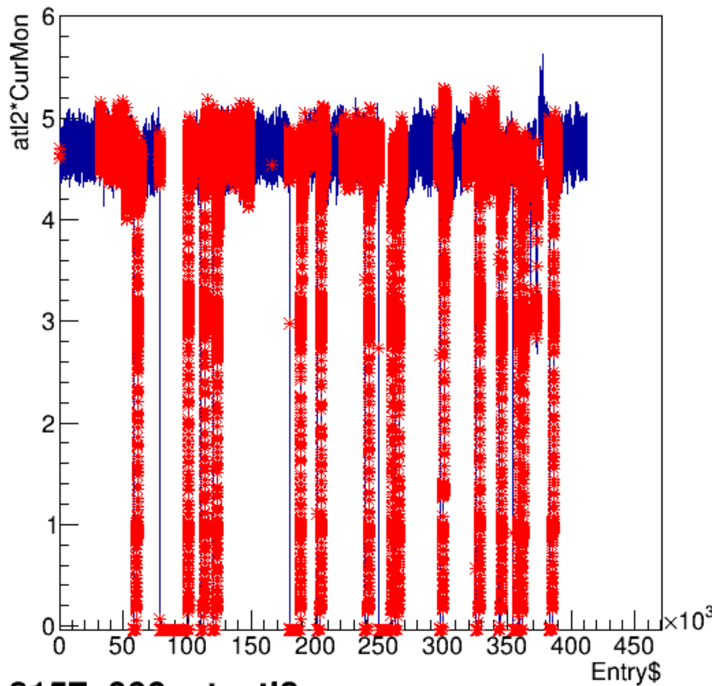
atl2*CurMon:Entry$
