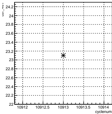
usr_4eY:cyclenum {run == 8245}
