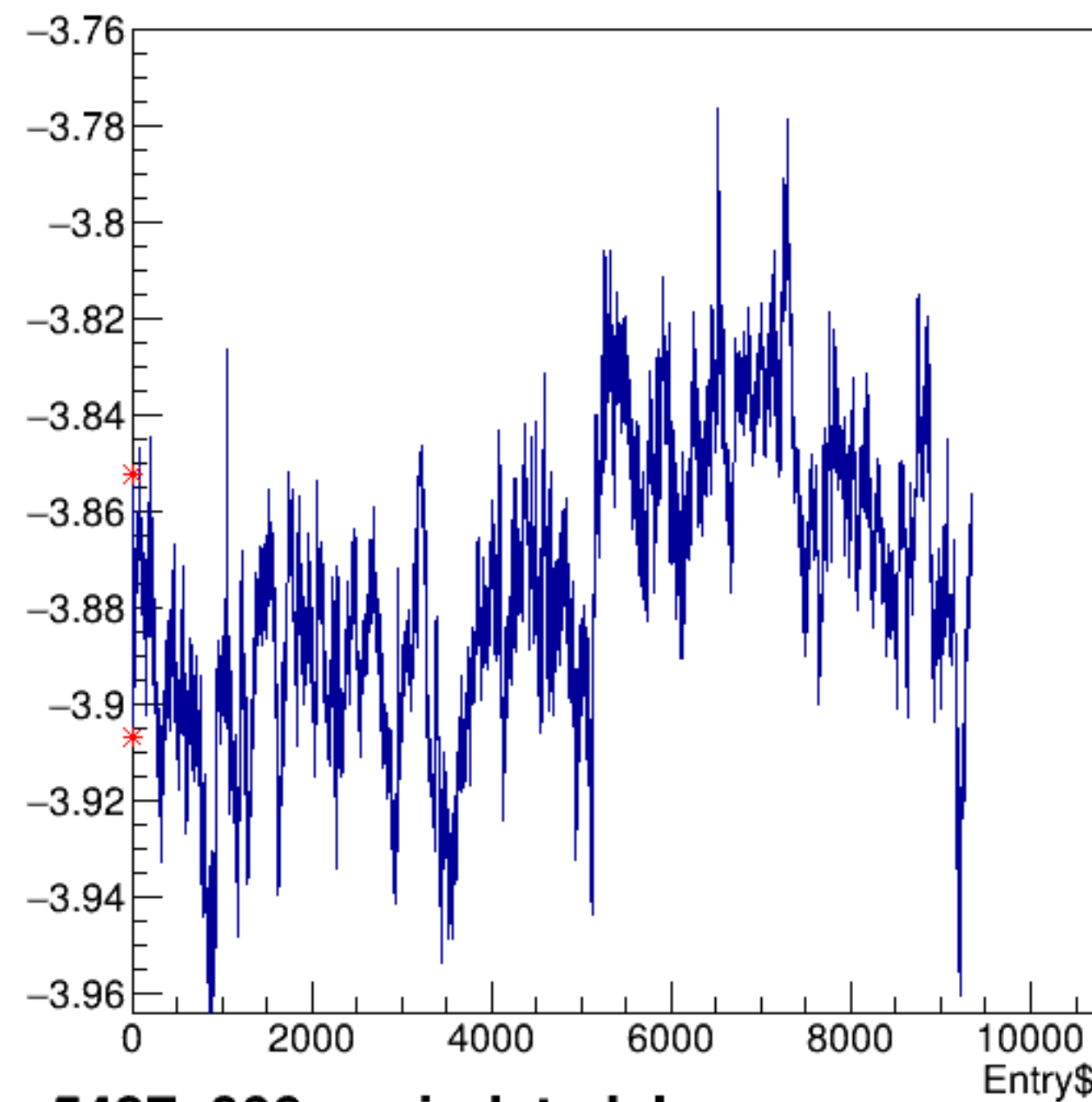
dsl*CurMon:Entry$
