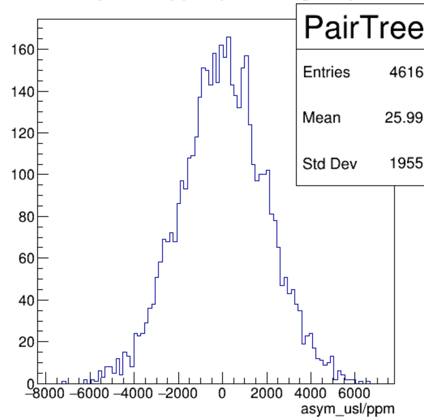
asym_usl/ppm {ErrorFlag==0}
