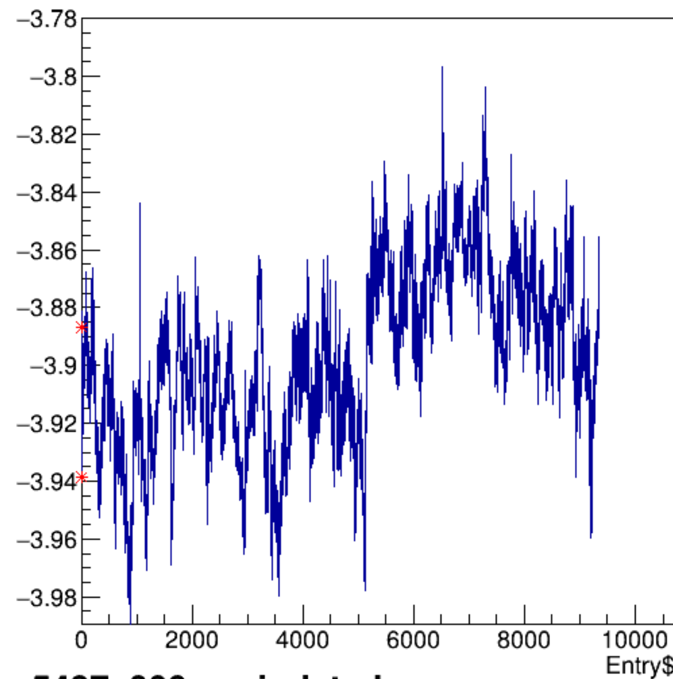
dsr*CurMon:Entry$
