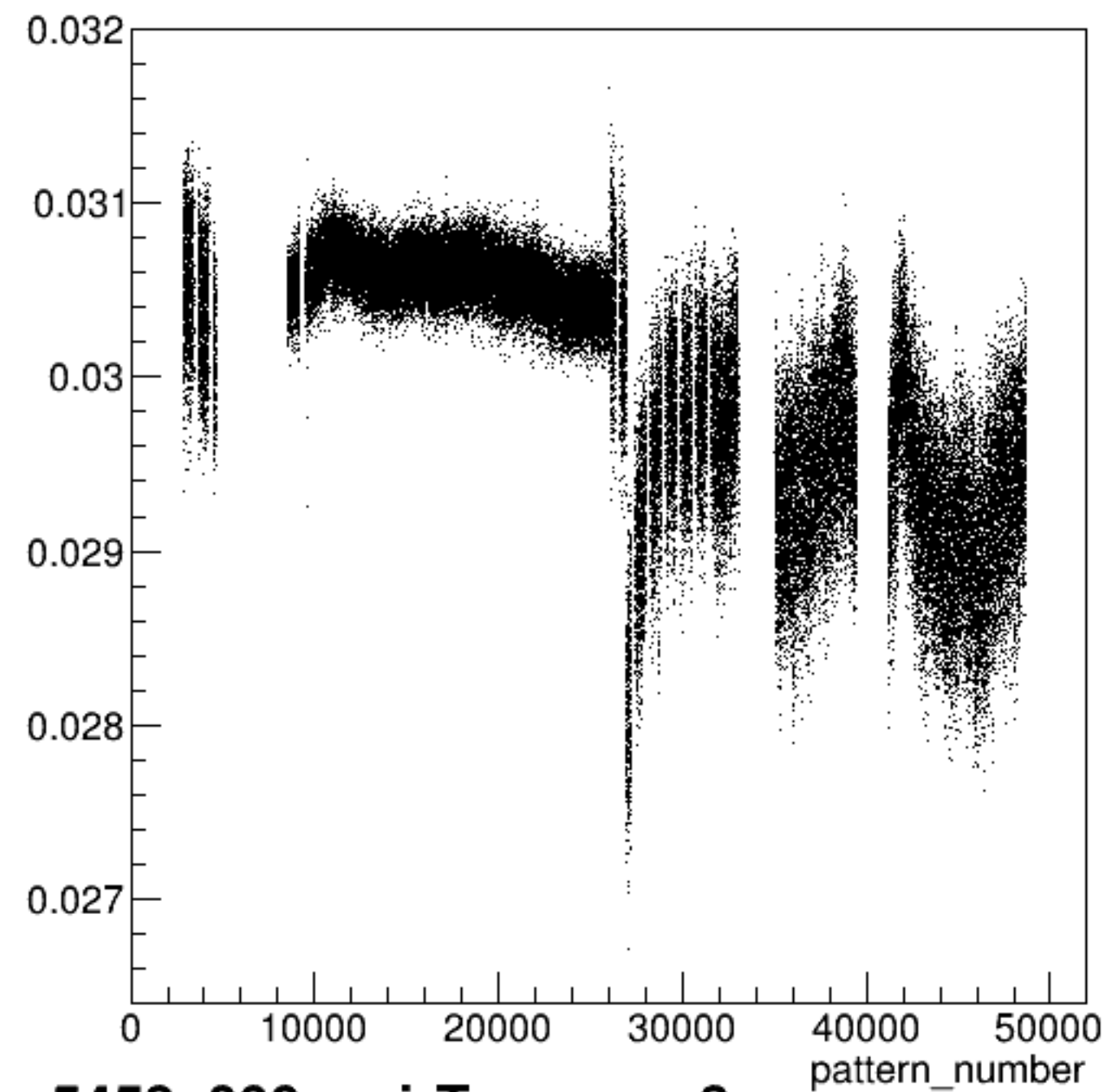
yield_sam3:pattern_number {ErrorFlag==0}
