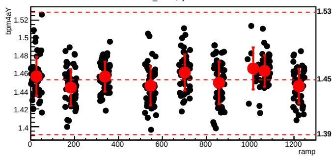
bmod_trim7,cyc=4130
