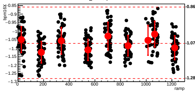
bmod_trim7,cyc=4130
