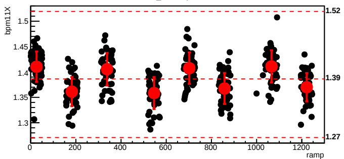
bmod_trim5,cyc=4130
