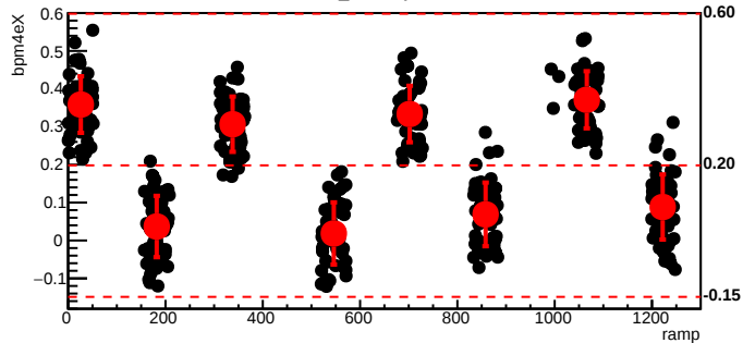
bmod_trim5,cyc=4130
