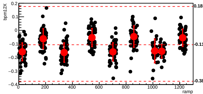
bmod_trim4,cyc=4130
