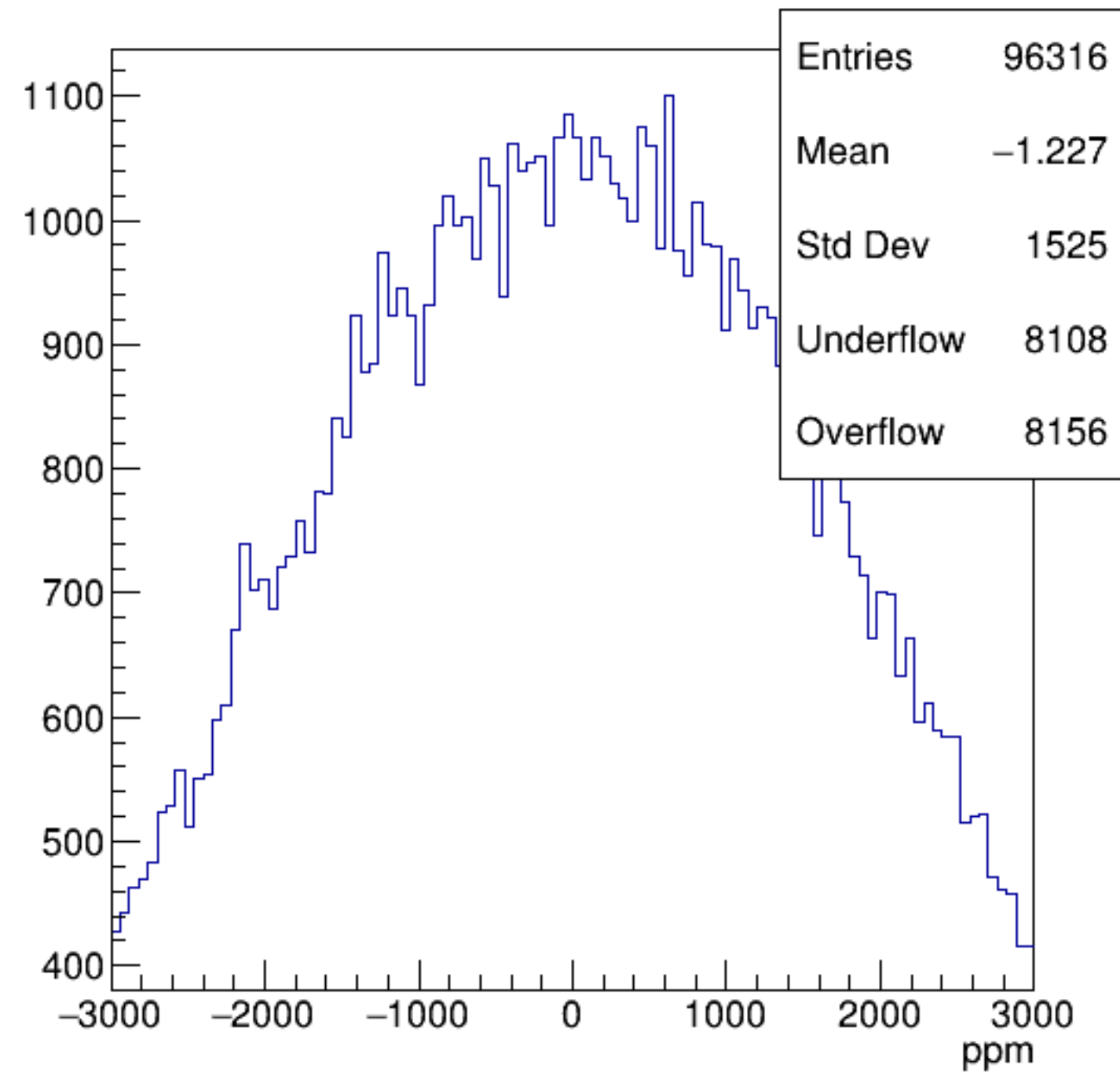
asym_sam4
