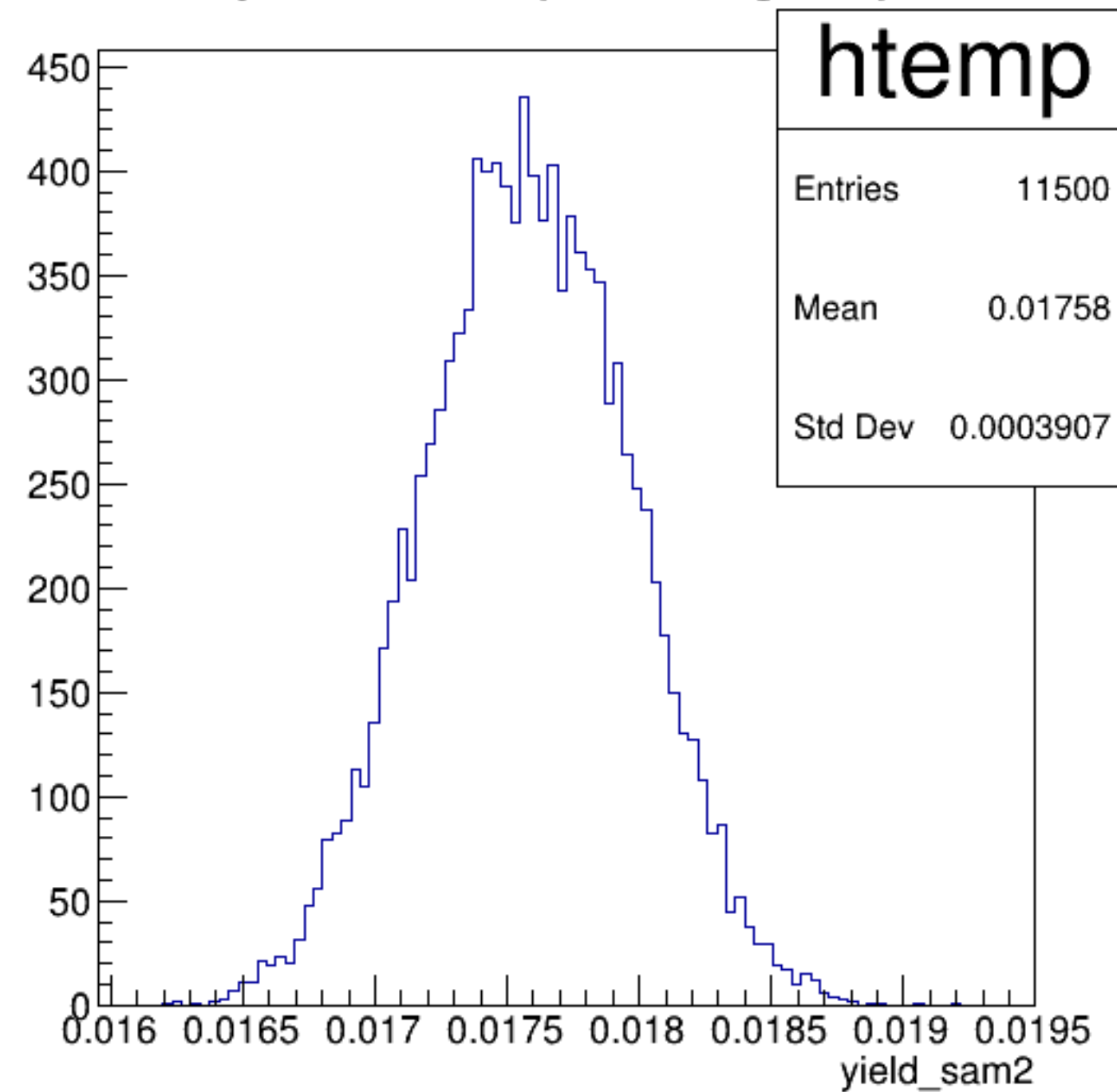
yield_sam2 {ErrorFlag==0}
