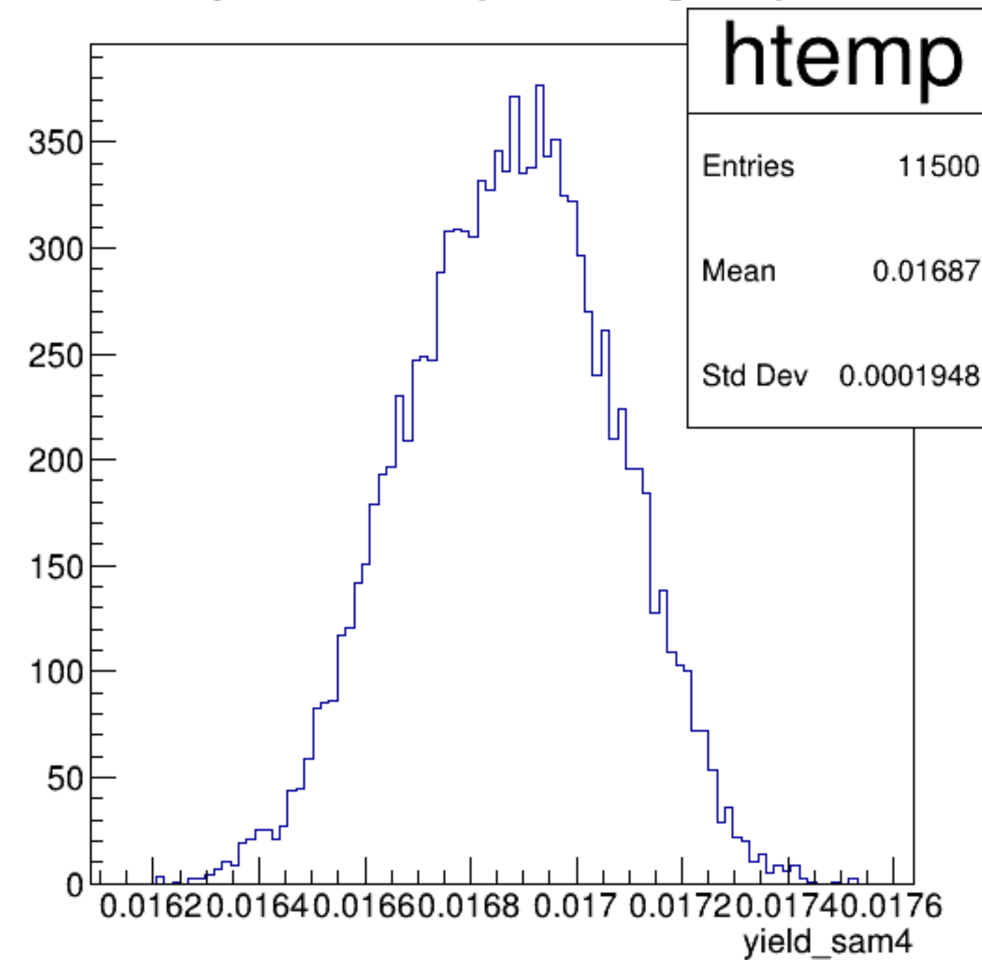
yield_sam4 {ErrorFlag==0}
