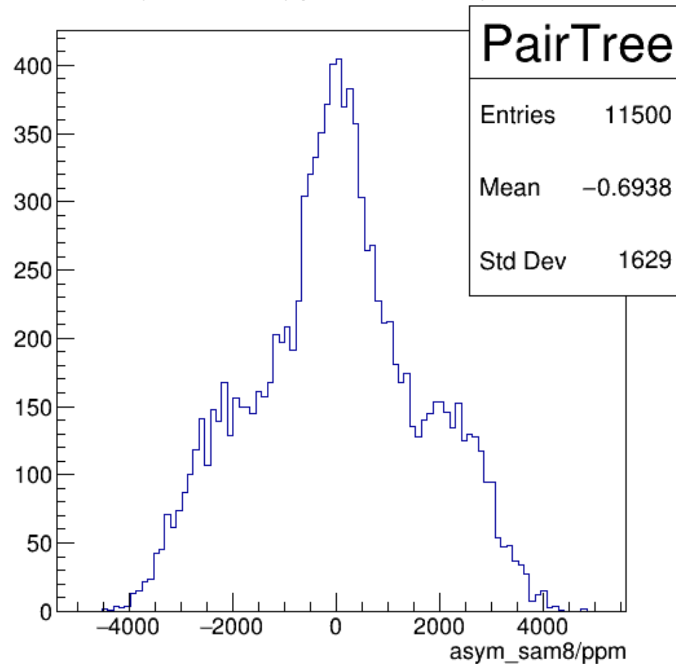
asym_sam8/ppm {ErrorFlag==0}
