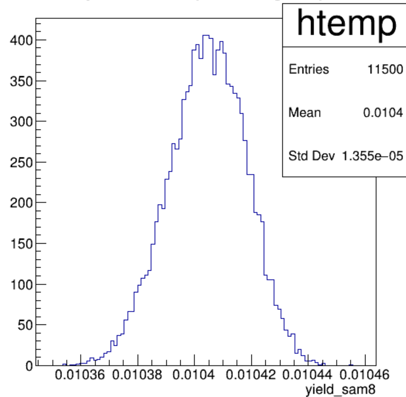
yield_sam8 {ErrorFlag==0}
