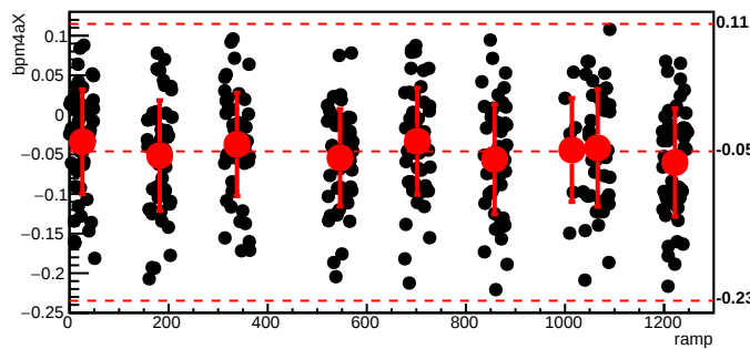
bmod_trim4,cyc=4230
