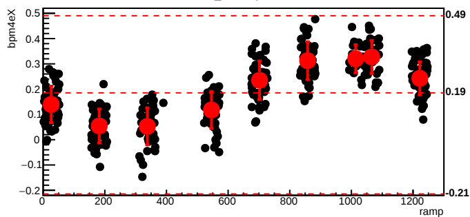
bmod_trim1,cyc=4230
