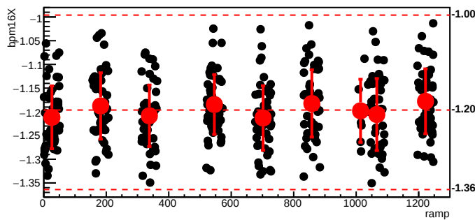
bmod_trim4,cyc=4230
