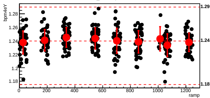
bmod_trim3,cyc=4230
