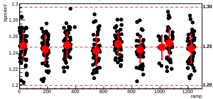
bmod_trim5,cyc=4230
