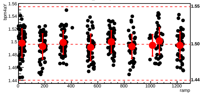
bmod_trim5,cyc=4230
