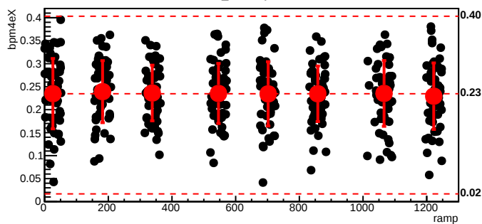
bmod_trim2,cyc=4230
