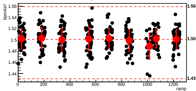
bmod_trim1,cyc=4230
