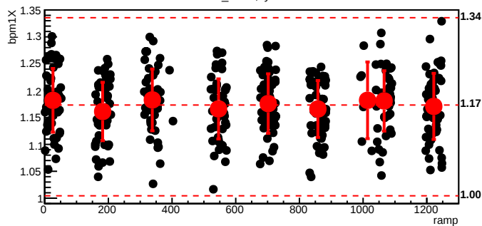
bmod_trim2,cyc=4298
