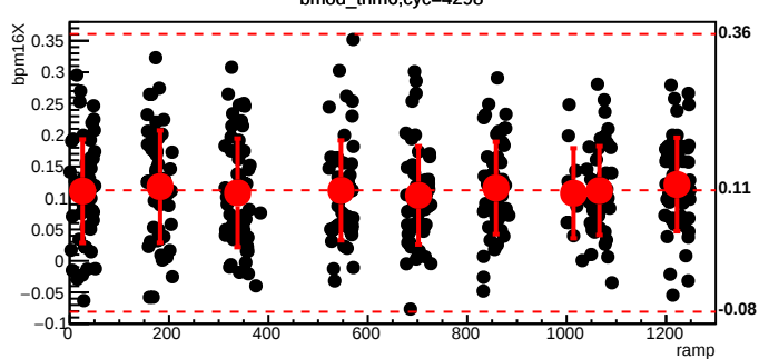
bmod_trim6,cyc=4298
