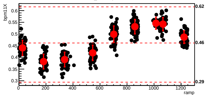
bmod_trim1,cyc=4298
