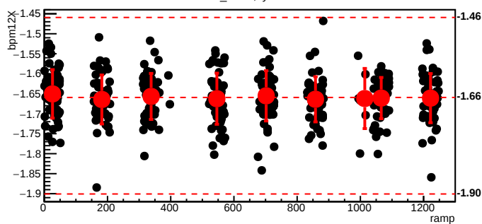
bmod_trim2,cyc=4298
