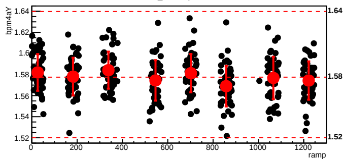
bmod_trim7,cyc=4298
