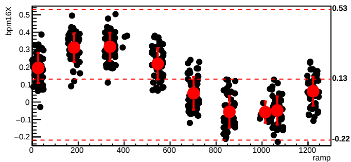
bmod_trim1,cyc=4298
