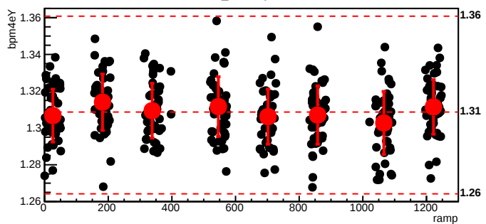
bmod_trim7,cyc=4298
