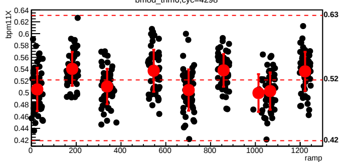
bmod_trim6,cyc=4298
