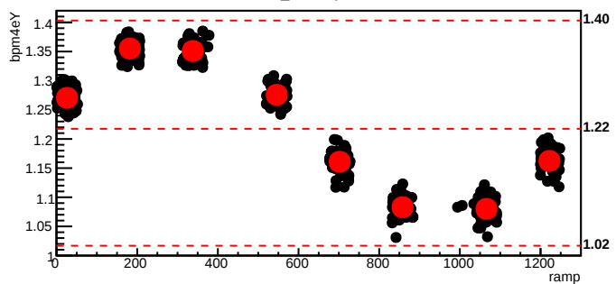
bmod_trim4,cyc=4298
