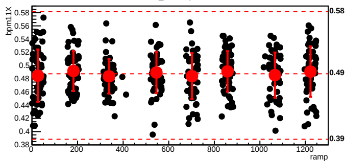
bmod_trim4,cyc=4298
