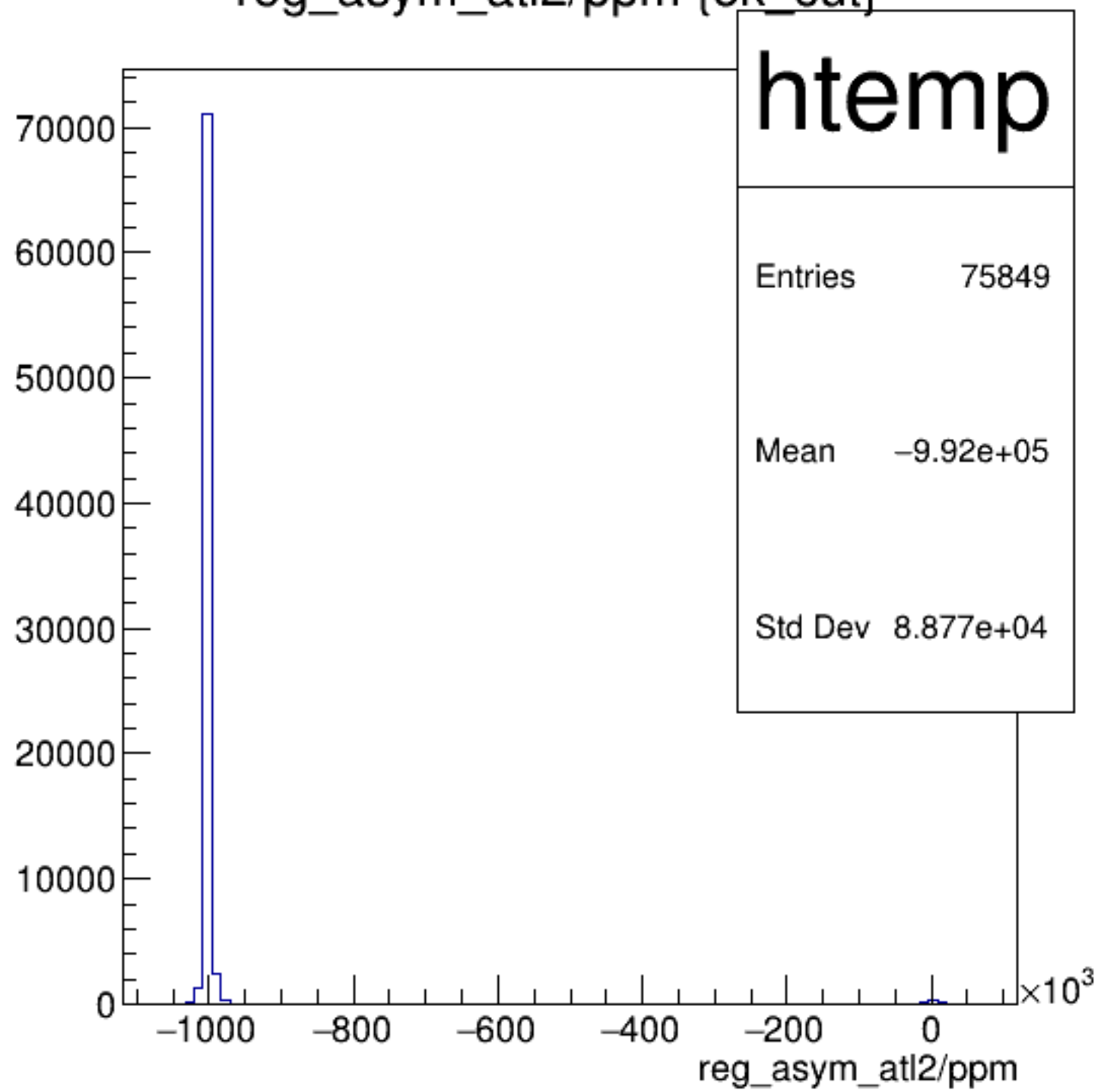
reg_asym_atl2/ppm {ok_cut}
