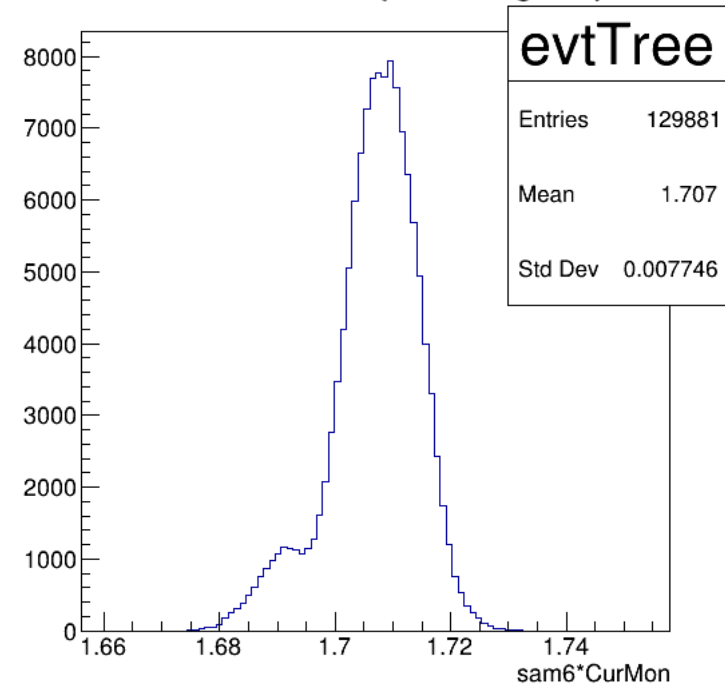
sam6*CurMon {ErrorFlag==0}
