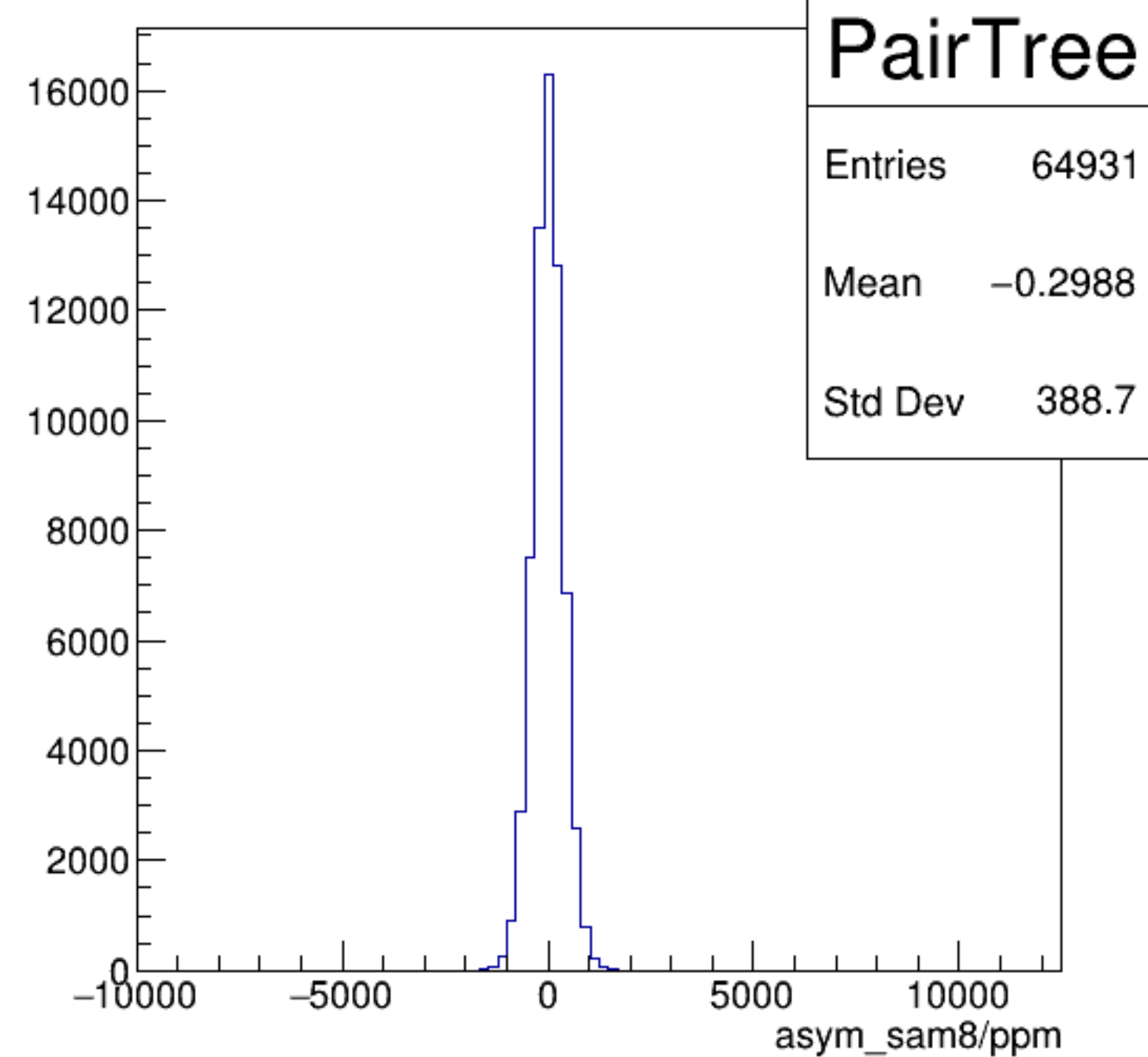
asym_sam8/ppm {ErrorFlag==0}
