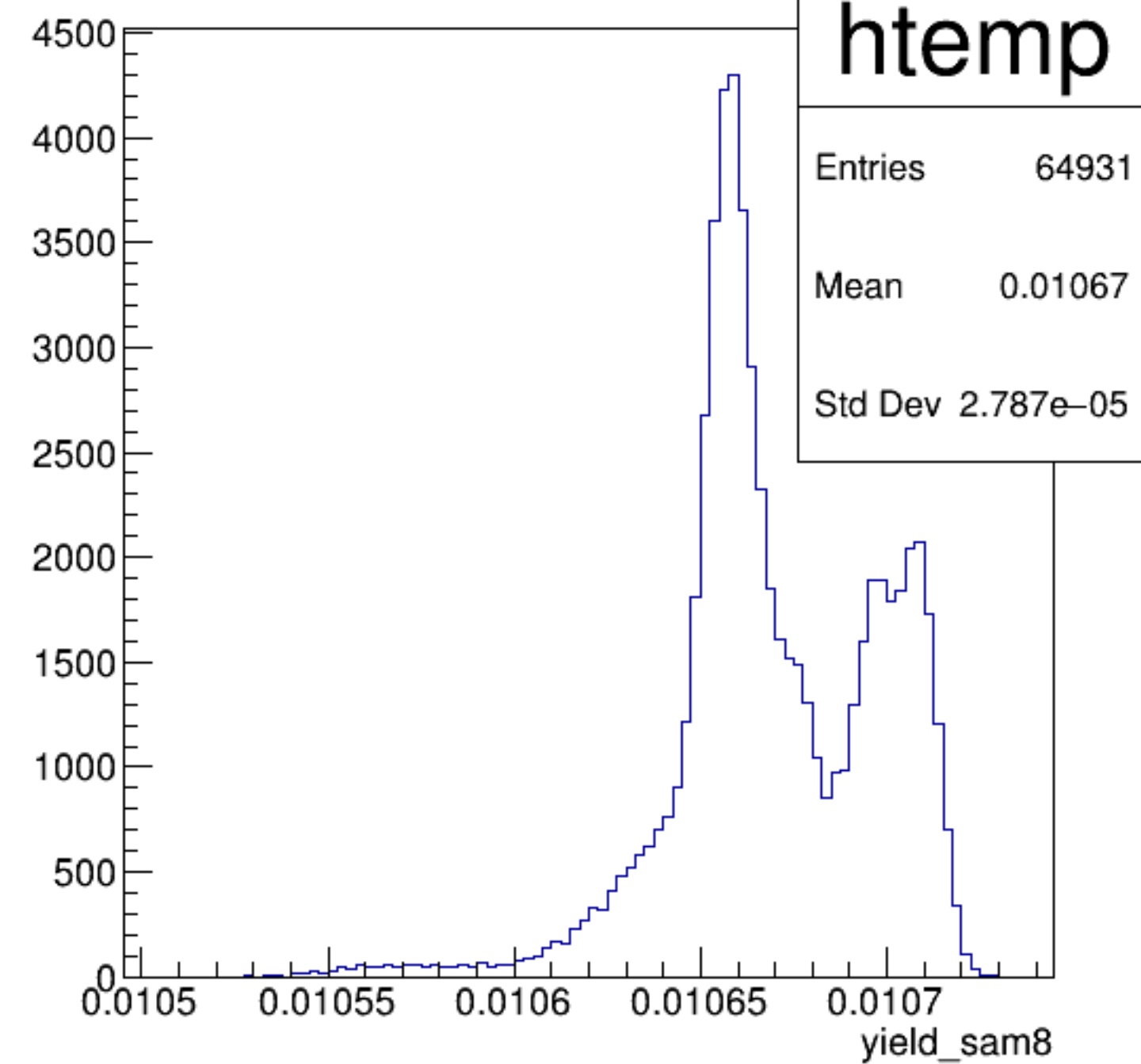
yield_sam8 {ErrorFlag==0}
