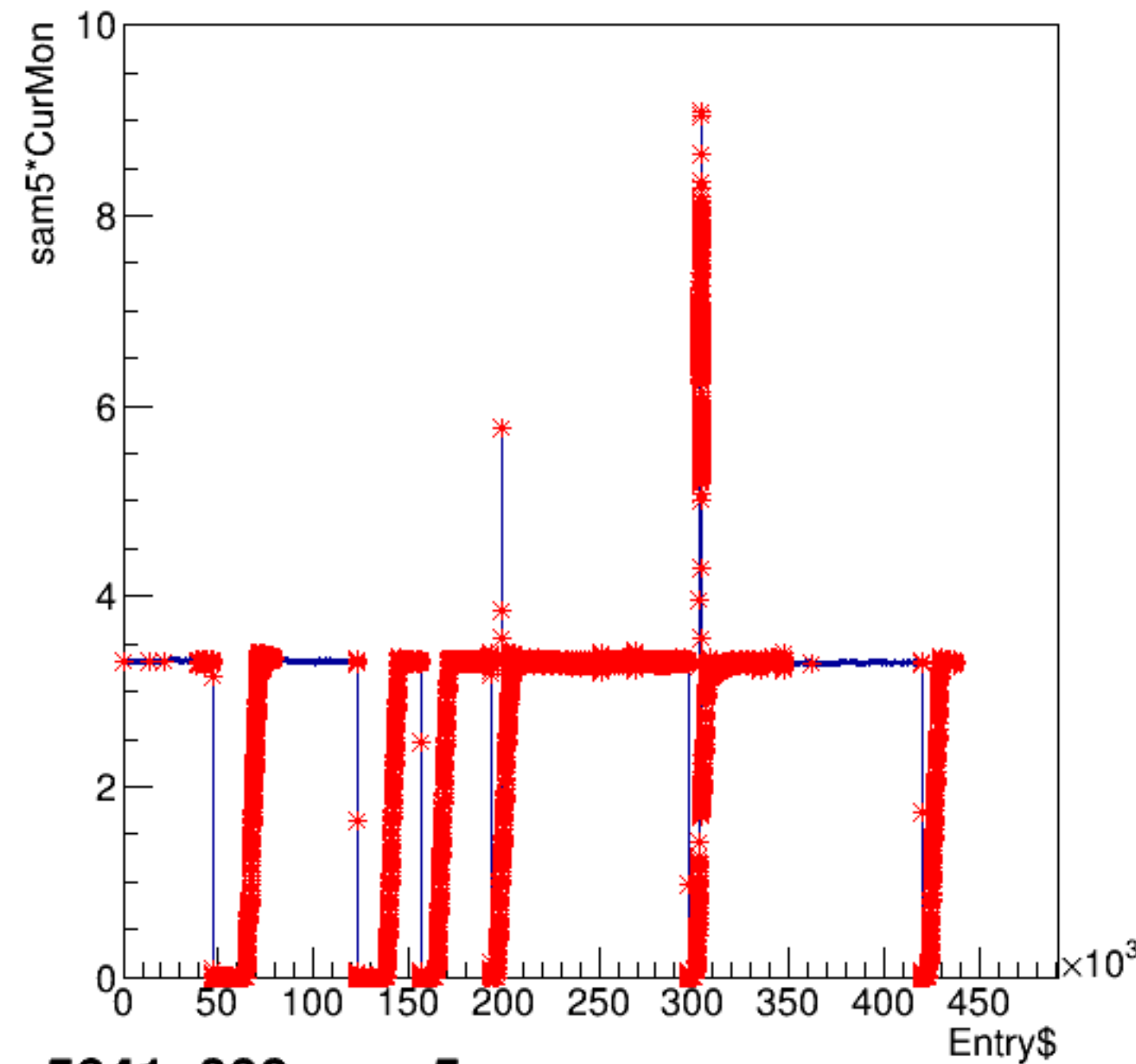
sam5*CurMon:Entry$
