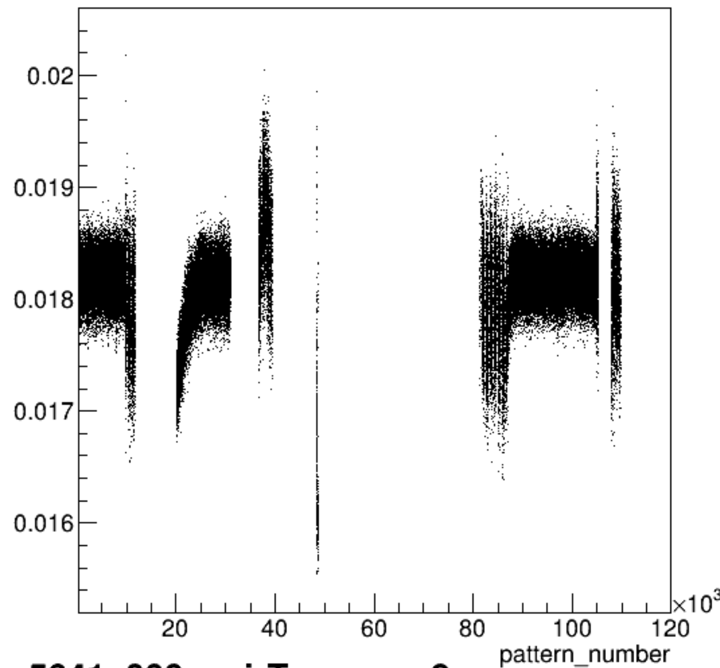
yield_sam2:pattern_number {ErrorFlag==0}
