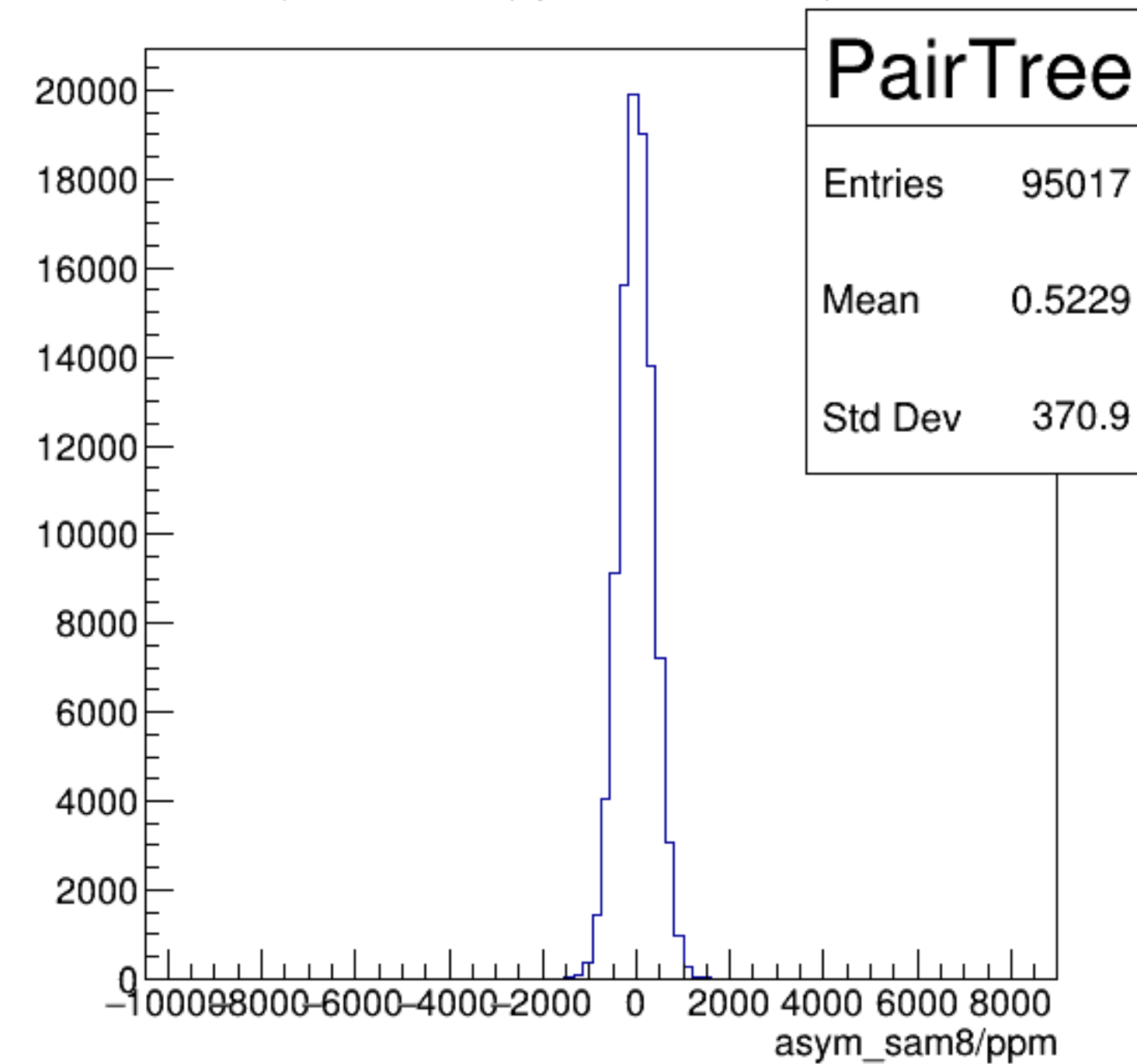
asym_sam8/ppm {ErrorFlag==0}
