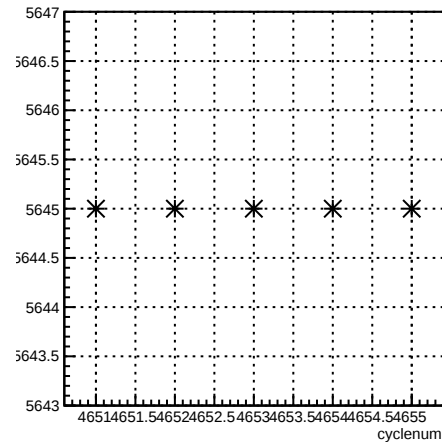
run:cyclenum {run == 5645}
