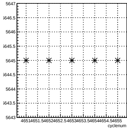
run:cyclenum {run == 5645}
